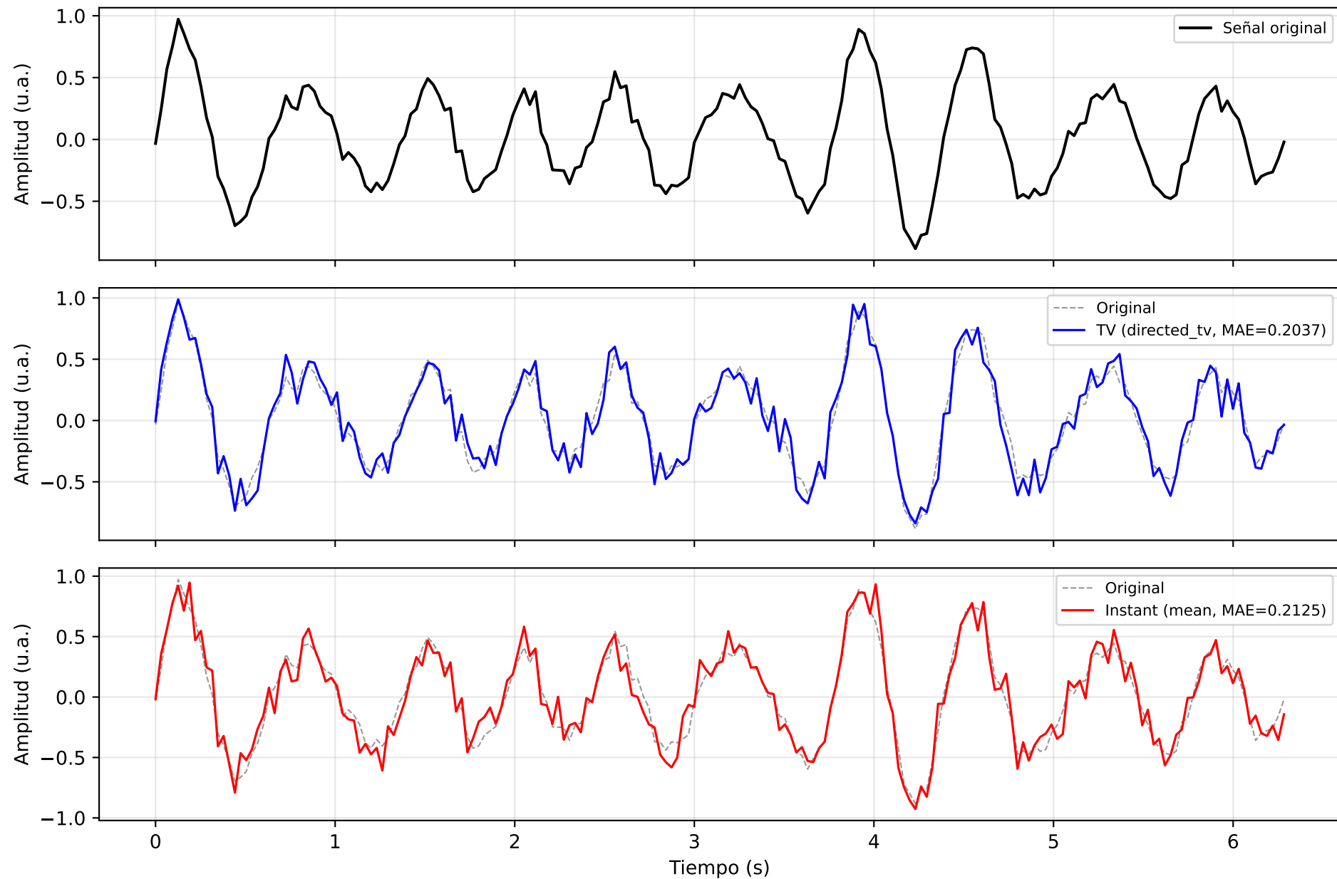
it20_synthetic_alpha_high_missing — Señal EEG: Original vs Reconstrucción
