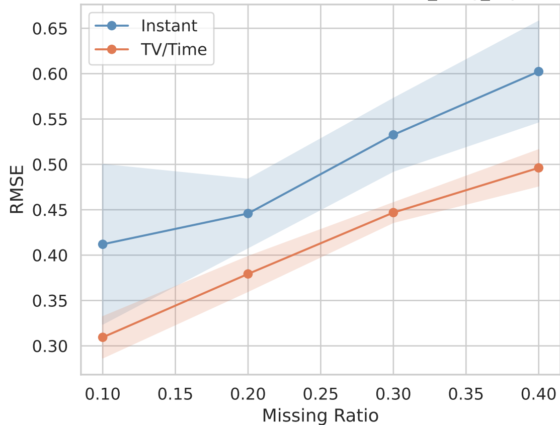
RMSE — TV/Time vs Instant — it23b_knng_3syn
