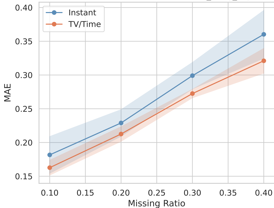
MAE — TV/Time vs Instant — it23b_knng_3syn
