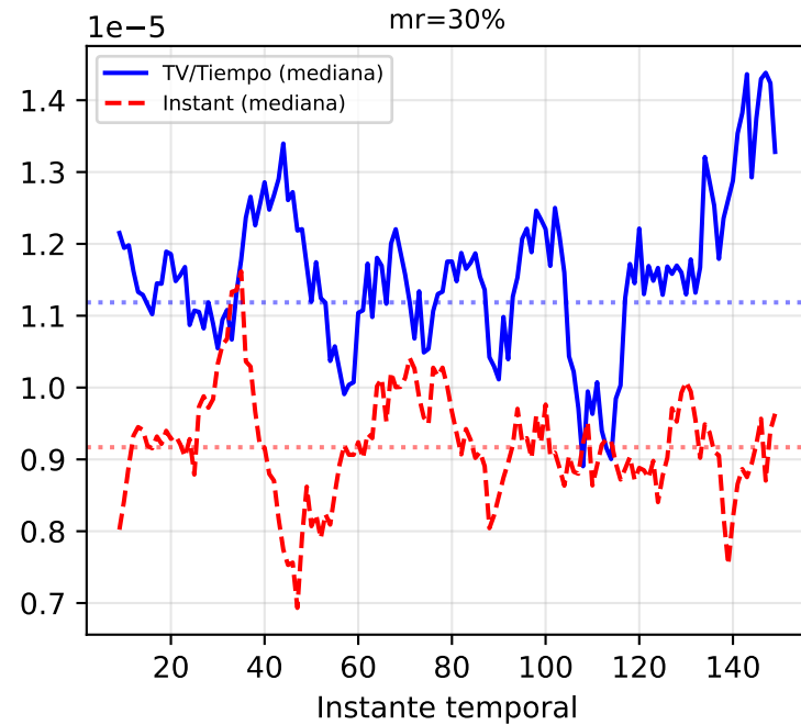
it24_physionet_all_scenarios — Error de Reconstrucción Temporal por Escenario
