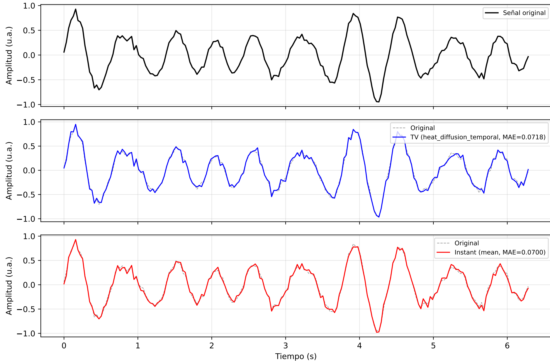
it28_nnk_3syn — Señal EEG: Original vs Reconstrucción
