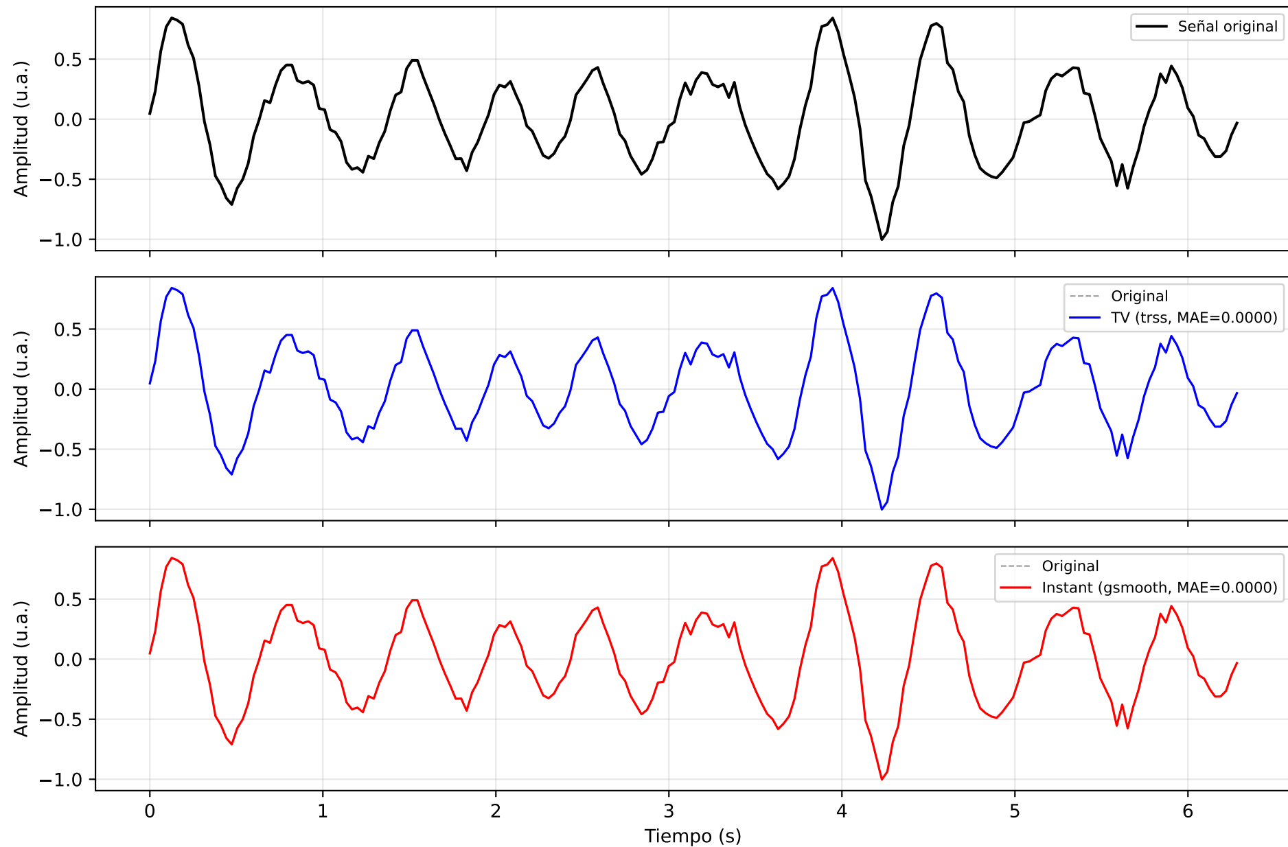
it44_physionet_allruns_allsubj — Señal EEG: Original vs Reconstrucción
