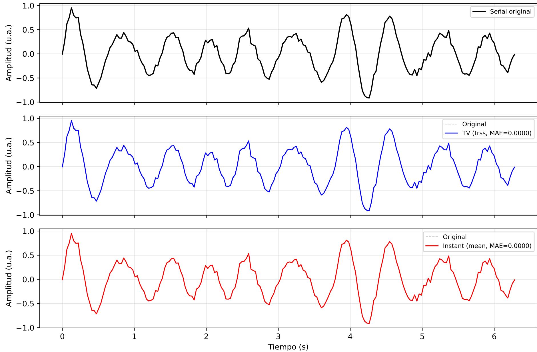
it64_bci_competition_single_subj — Señal EEG: Original vs Reconstrucción
