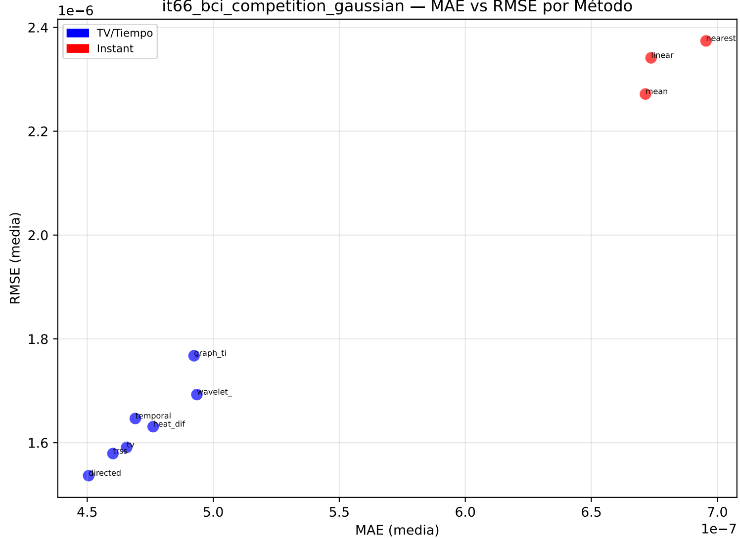
it66_bci_competition_gaussian — MAE vs RMSE por Método
