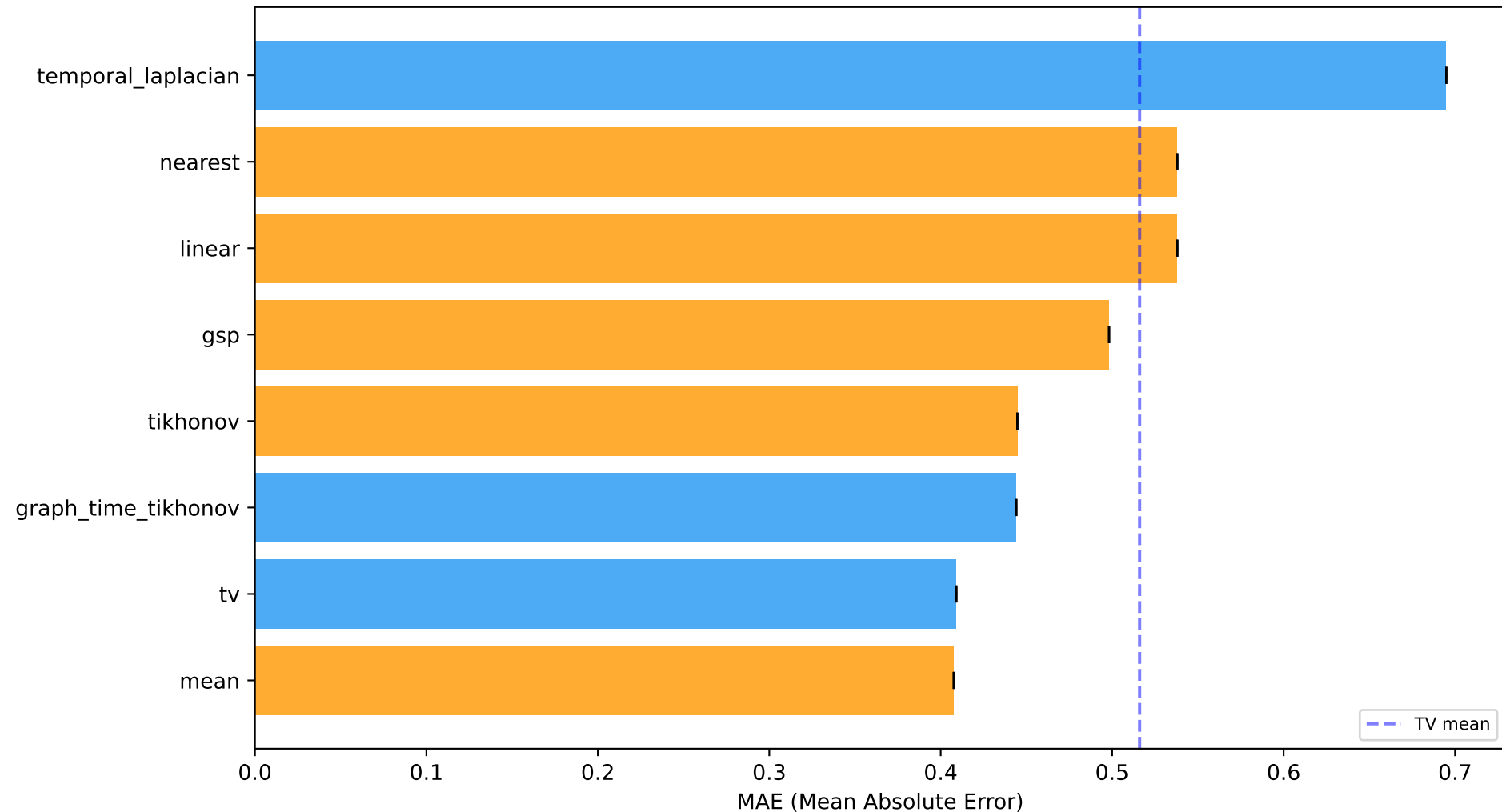
it72_few_missing_2ch_synthetic MAE por Método (azul=TV, naranja=Instante)
