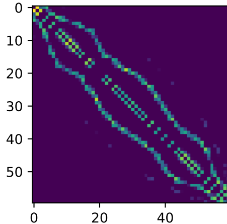
Kaliofolias
