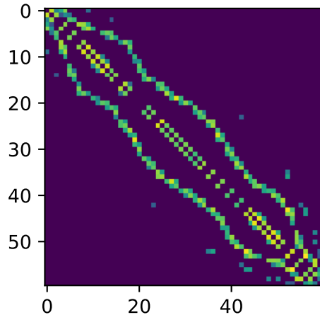
Sklearn KNN
