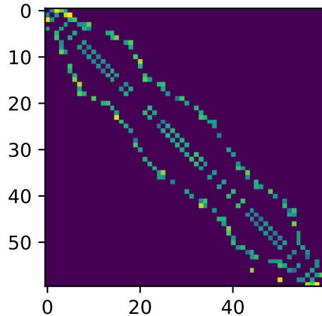
VKNN
