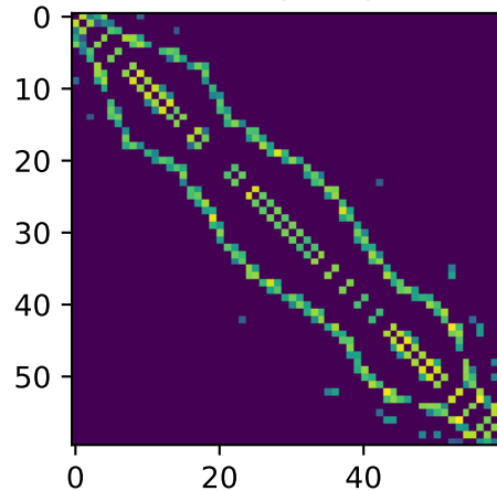
KNN(NNK)
