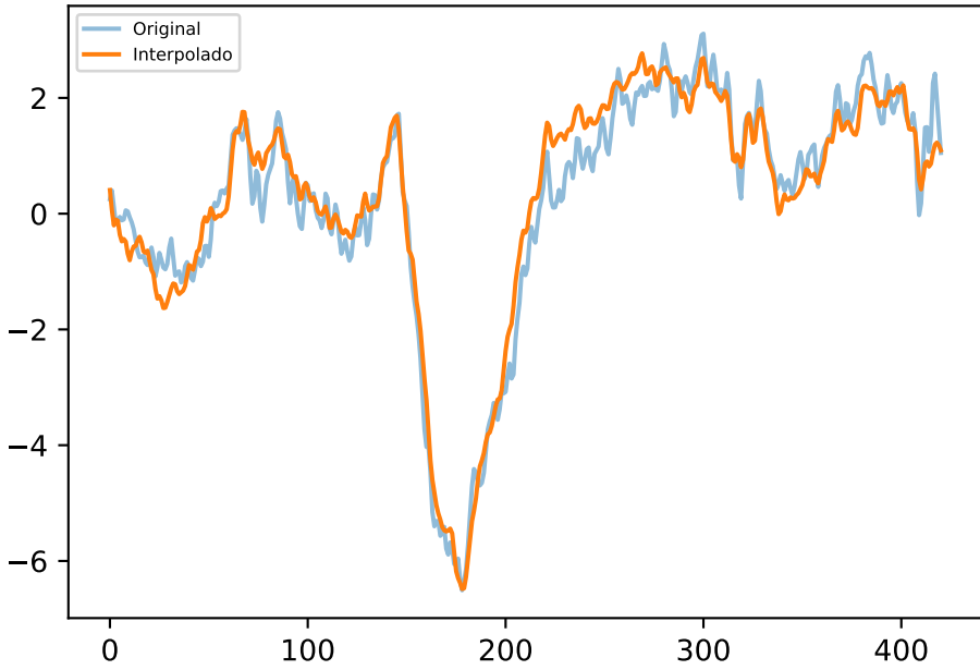
NNI
