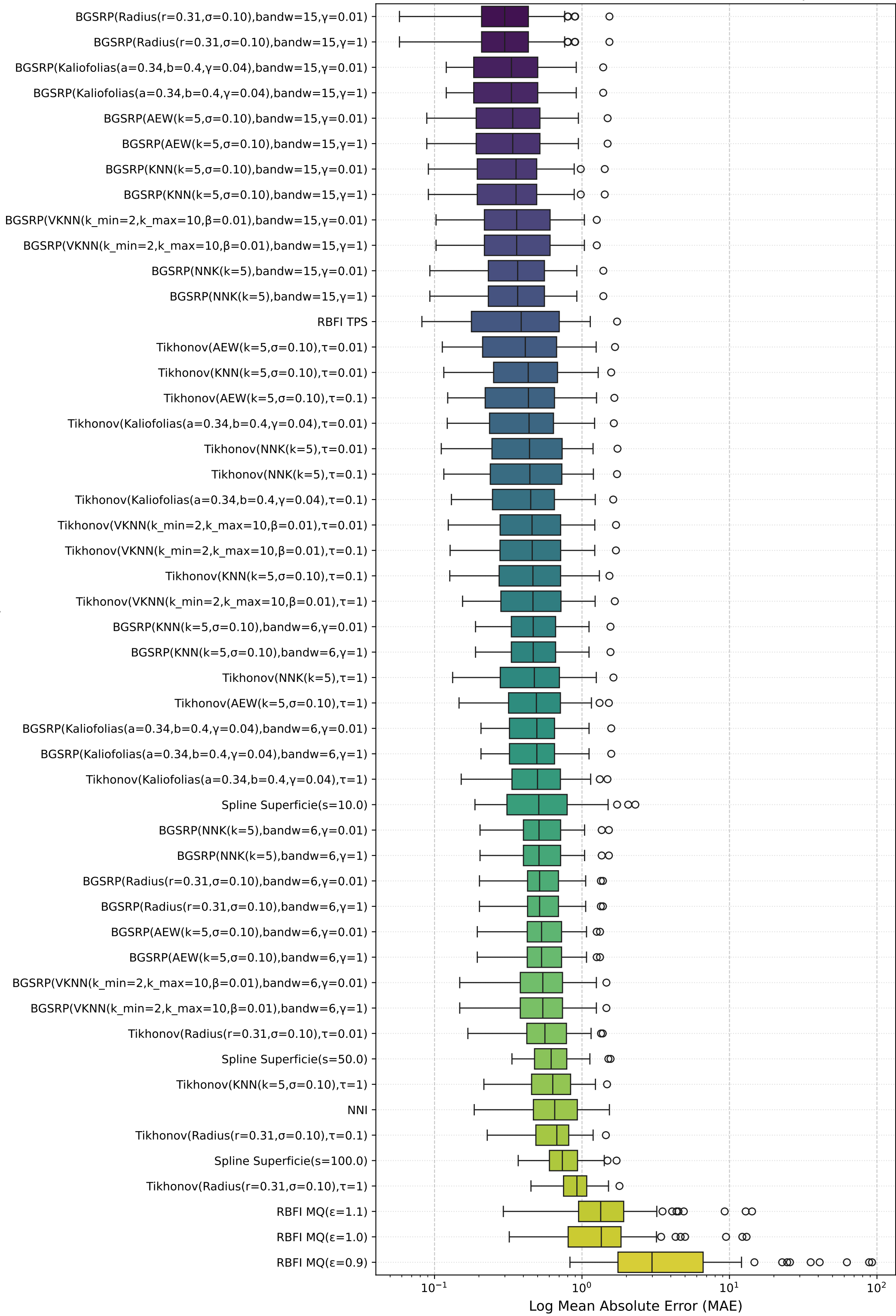
Distribución de MAE (N=60 escenarios) - Boxplot
