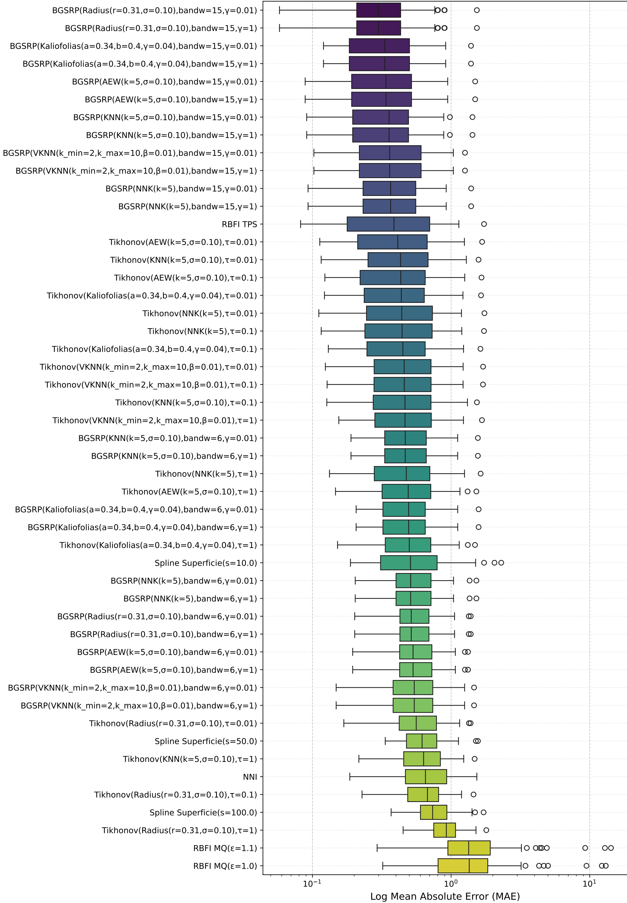
Distribución de MAE (N=60 escenarios) - Boxplot
