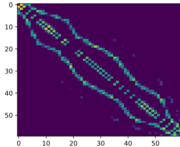
Kaliofolias
