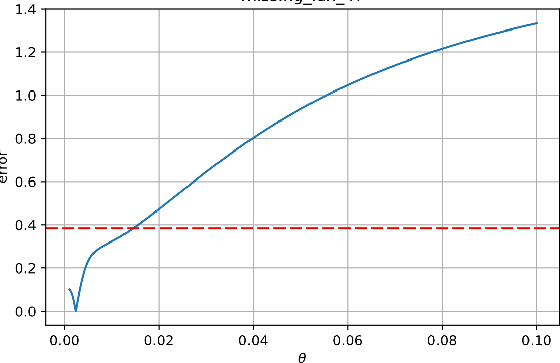
missing_idx_47
