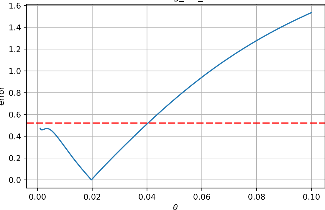
missing_idx_3
