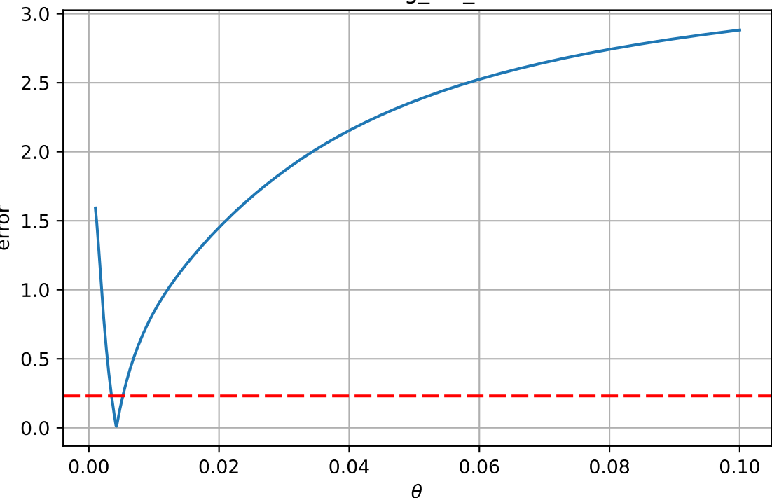
missing_idx_28
