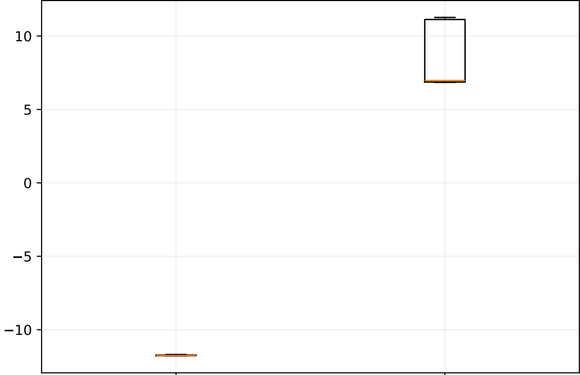
SNR
