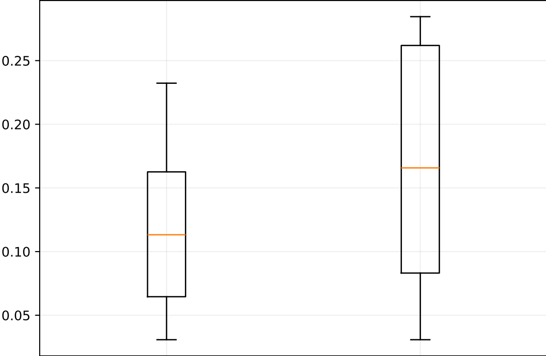
MAE
