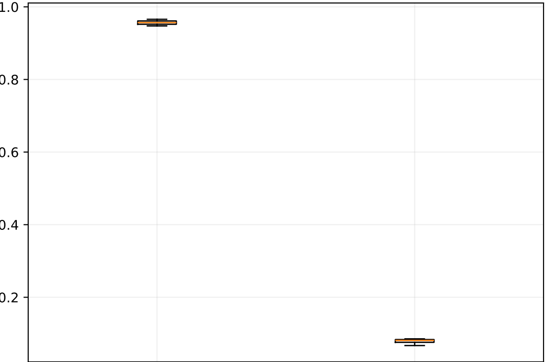
MAE
