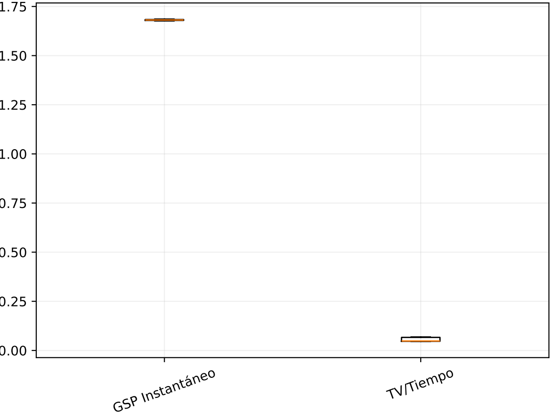
MAE
