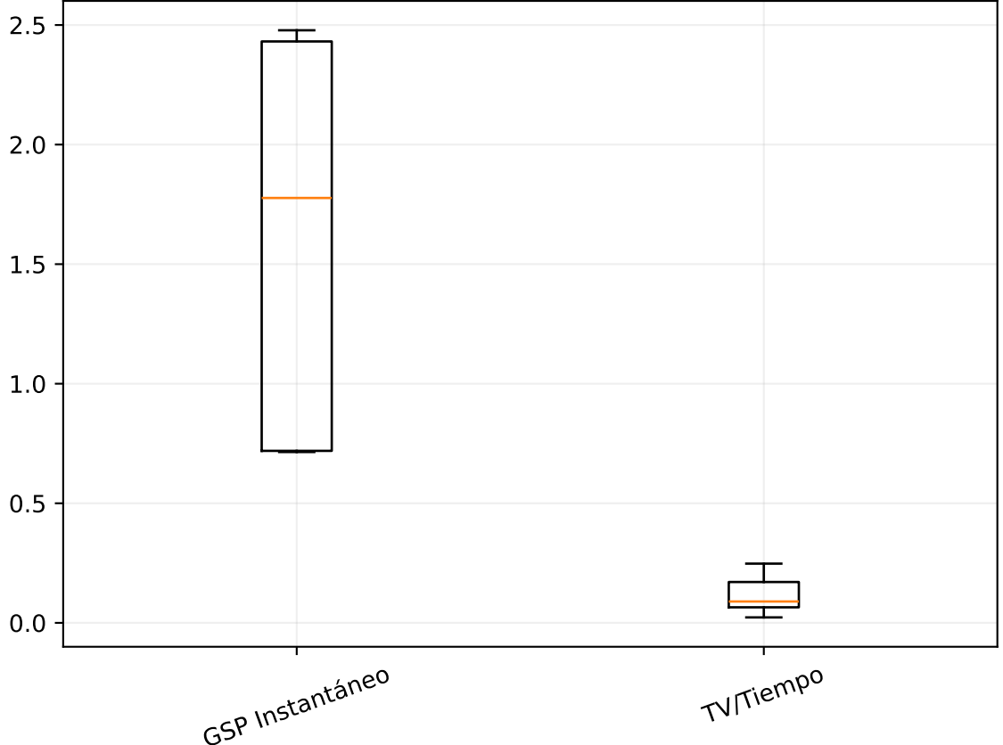
MAE
