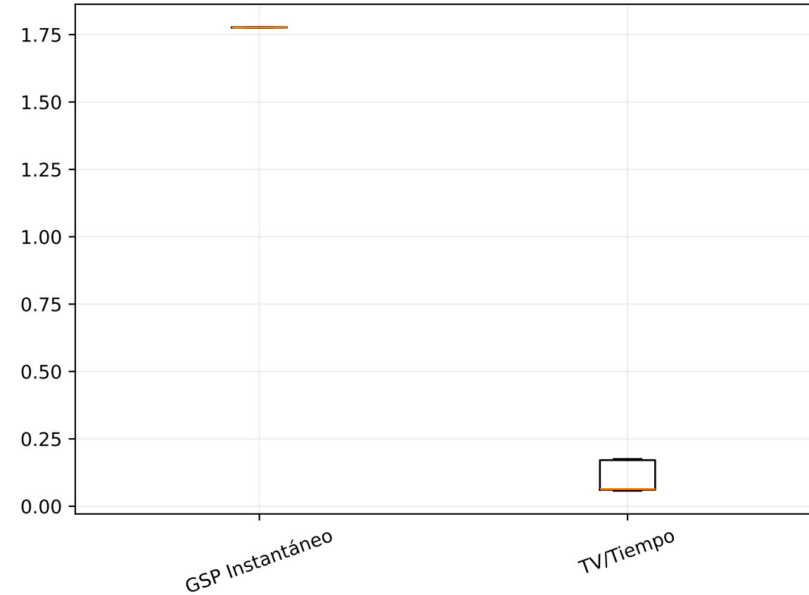
MAE
