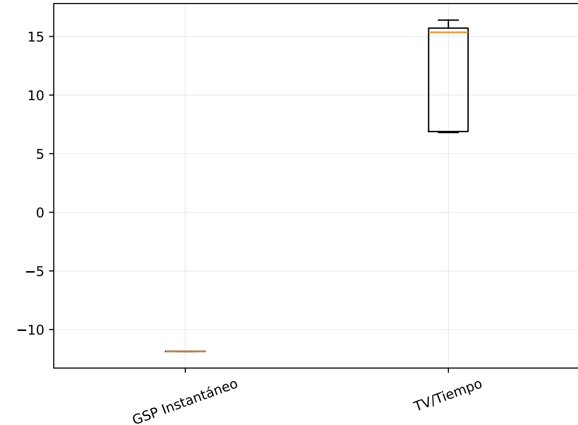
SNR
