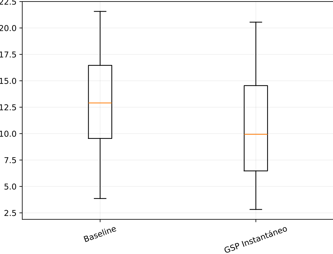
SNR
