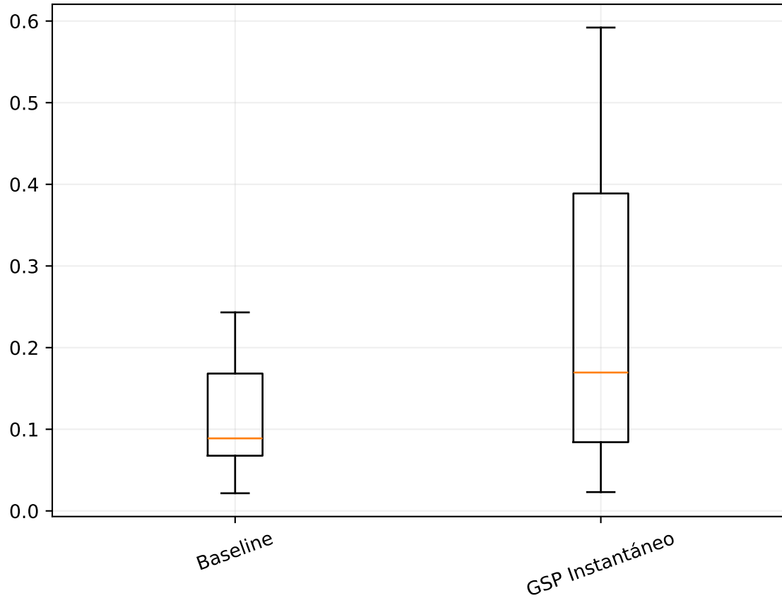
MAE
