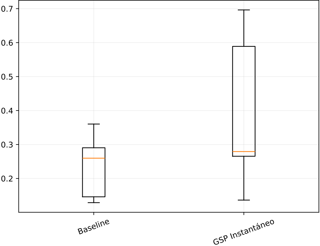
SNR
