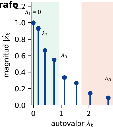
(b) Espectro del Laplaciano
