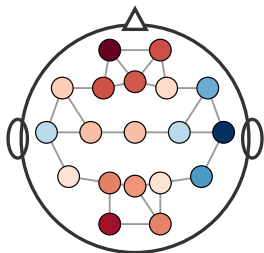
(a) EEG como grafo
