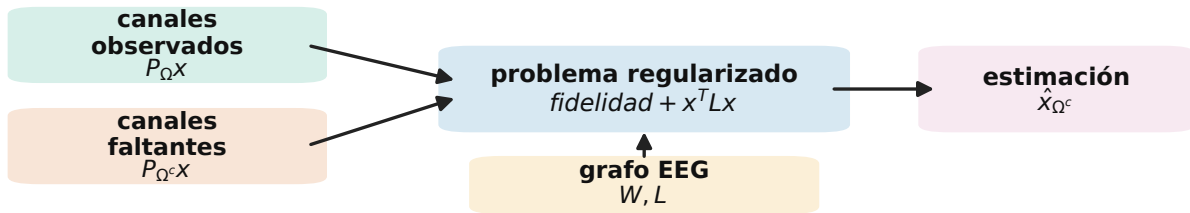
(c) Reconstrucción regularizada
