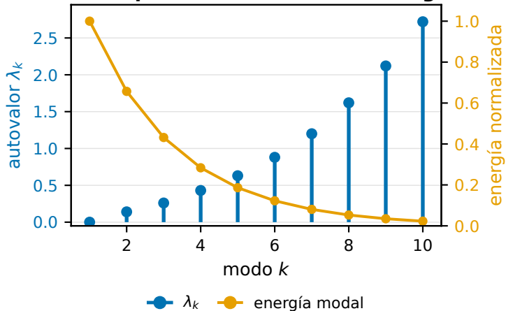
(b) Espectro: autovalor vs. energía
