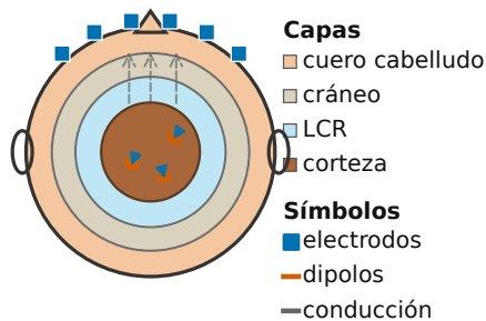
(a) Origen cortical y conducción
