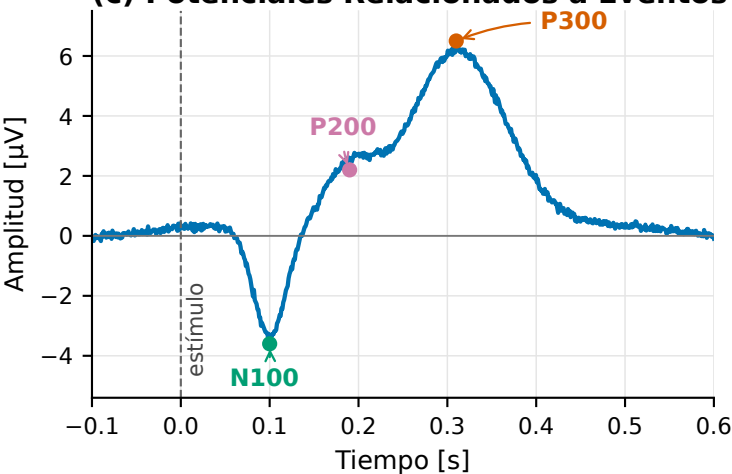
(c) Potenciales Relacionados a Eventos (ERP)
