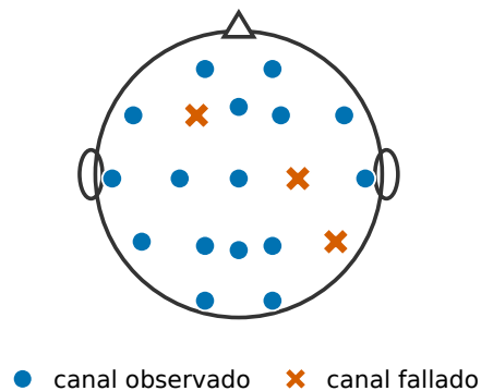
(d) Topografía: canales buenos y fallados
