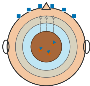
(a) Origen cortical y conducción
