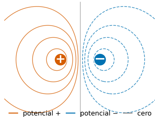
(b) Campo del dipolo
