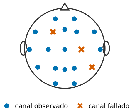
(d) Topografía: canales buenos y fallados
