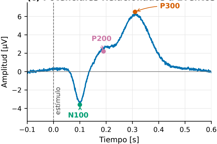
(c) Potenciales Relacionados a Eventos (ERP)
