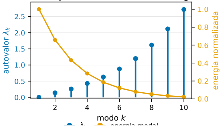
(b) Espectro: autovalor vs. energía
