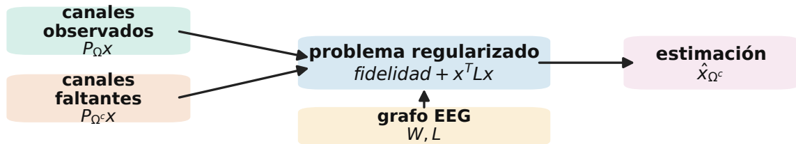
(c) Reconstrucción regularizada
