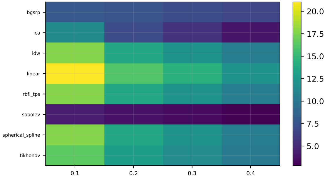
SNR heatmap
