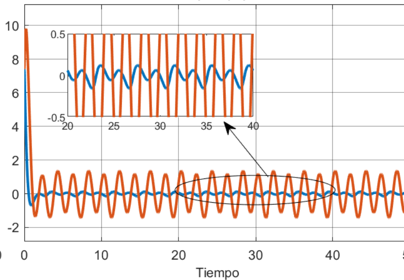
Error Brazo 4
