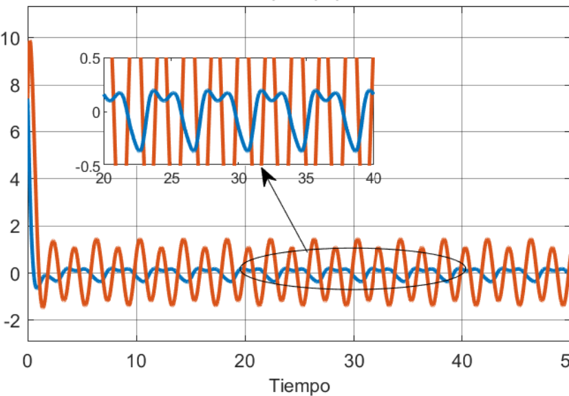
Error Brazo 2
