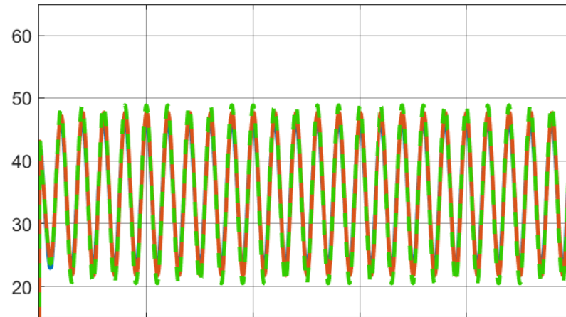
Fuerza Brazo 3
