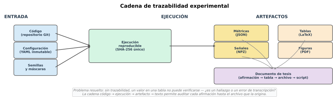
Figura 3.3: Cadena de trazabilidad experimental. Cada afirmación cuantitativa puede rastrearse desde el texto hasta una tabla o figura, desde allí al archivo JSON/CSV correspondiente y finalmente al script que generó el resultado.
