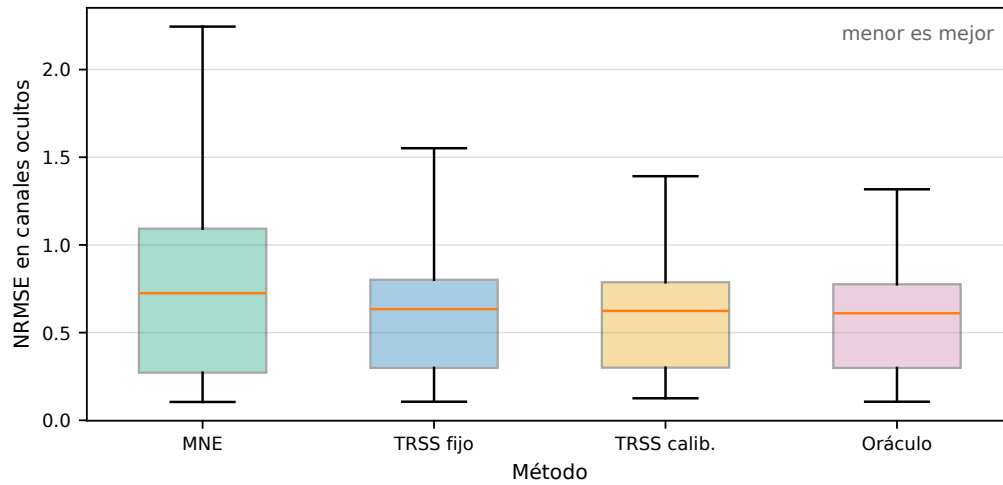
Figura 4.3: Distribución de NRMSE en la evaluación confirmatoria balanceada. La figura complementa la comparación mediana de la Tabla 4.4: TRSS desplaza la distribución hacia menor error relativo, pero la superposición entre cajas muestra que la mejora no es uniforme en todos los estratos.
