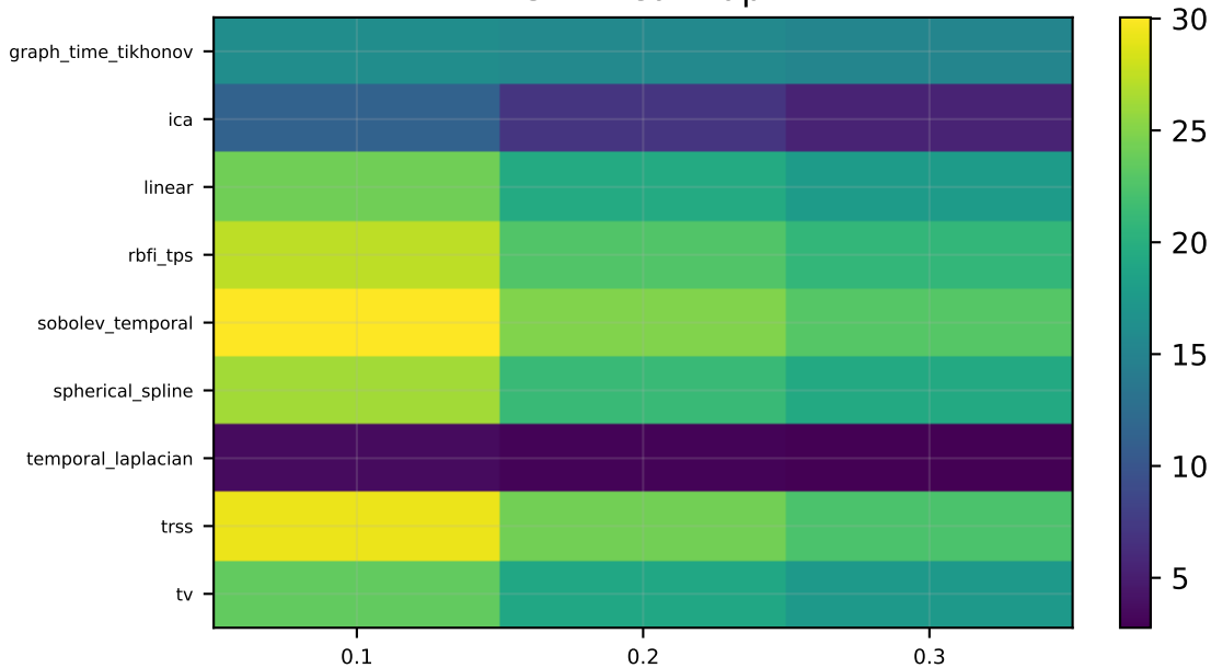
SNR heatmap
