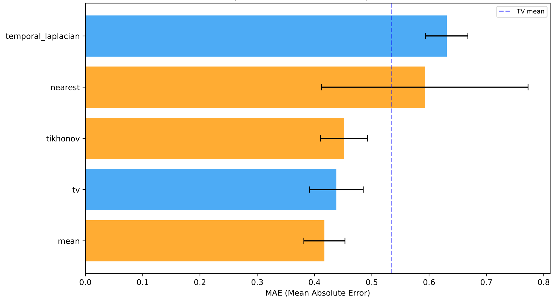
it75_few_missing_multi_synthetic MAE por Método (azul=TV, naranja=Instante)
