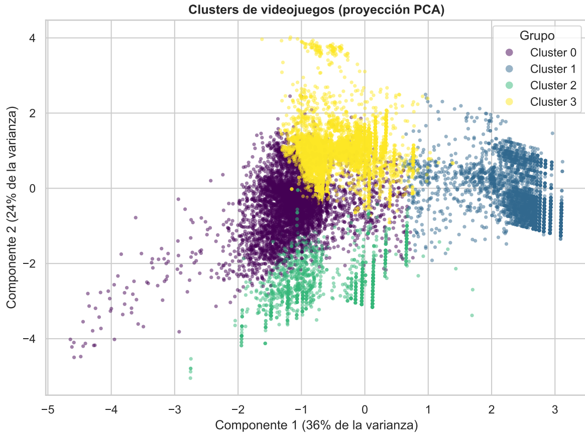
Figure 7: Clusters en 2 dimensiones (PCA)
