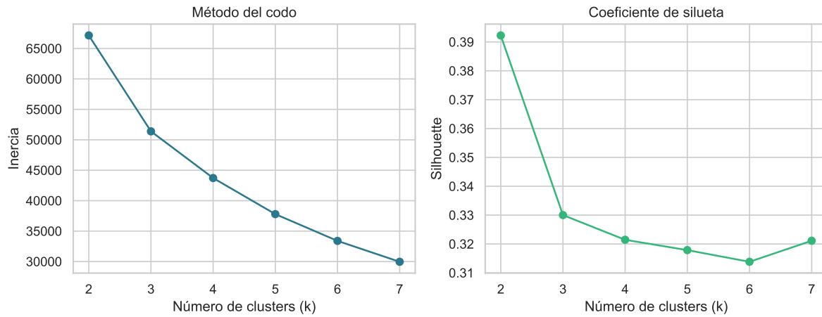
Figure 6: Selección de k
