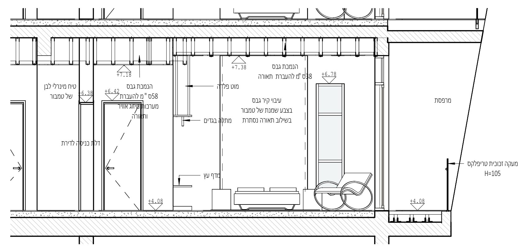
פריסת חדר מבט למיטה 1 : 50
