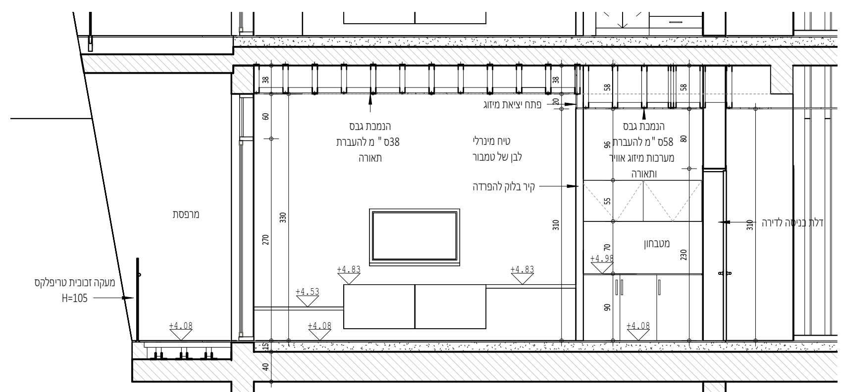
פריסה קיר טלוויזיה 1 : 50
