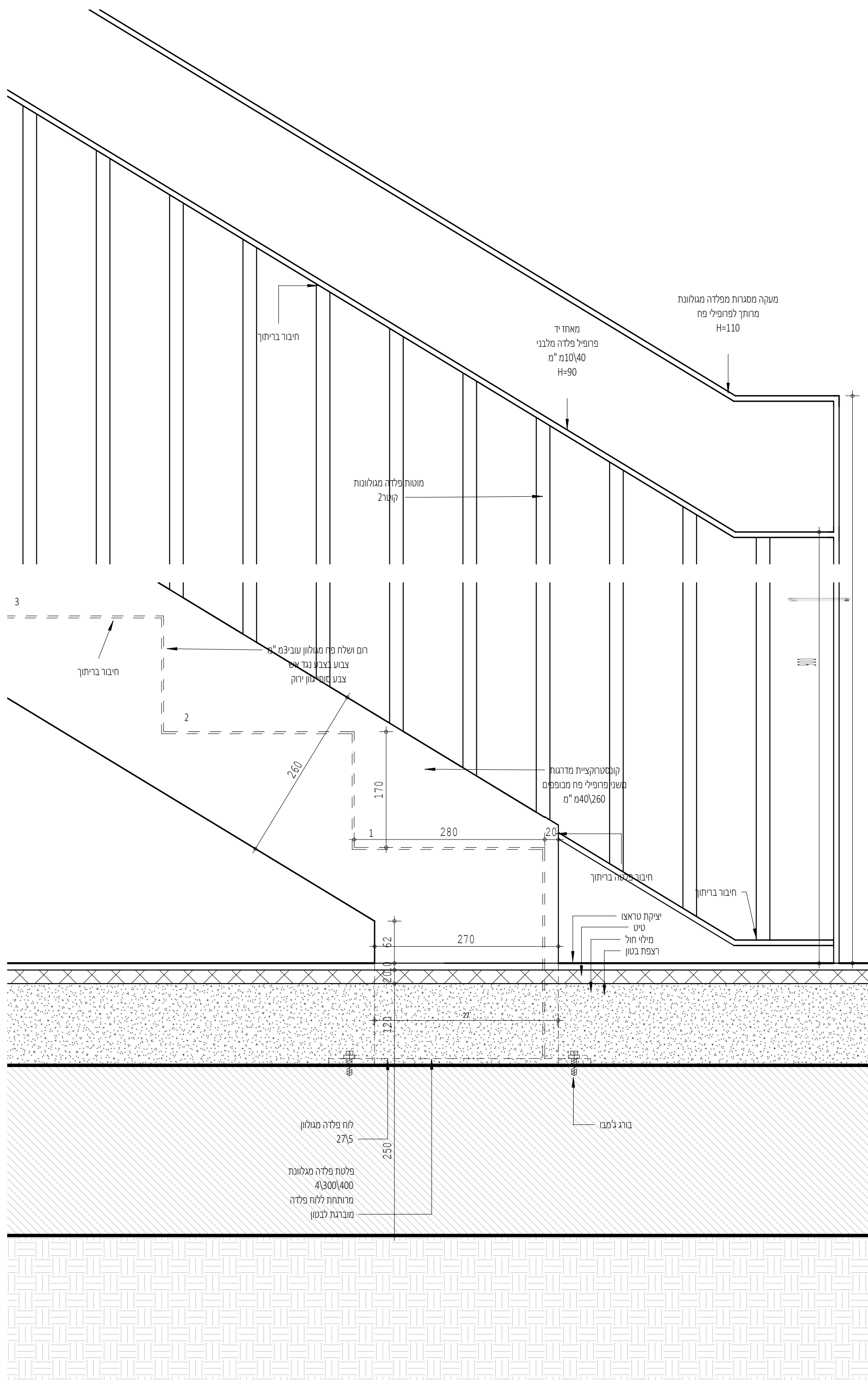
פרט מדרגות ראשונות 1 : 5
