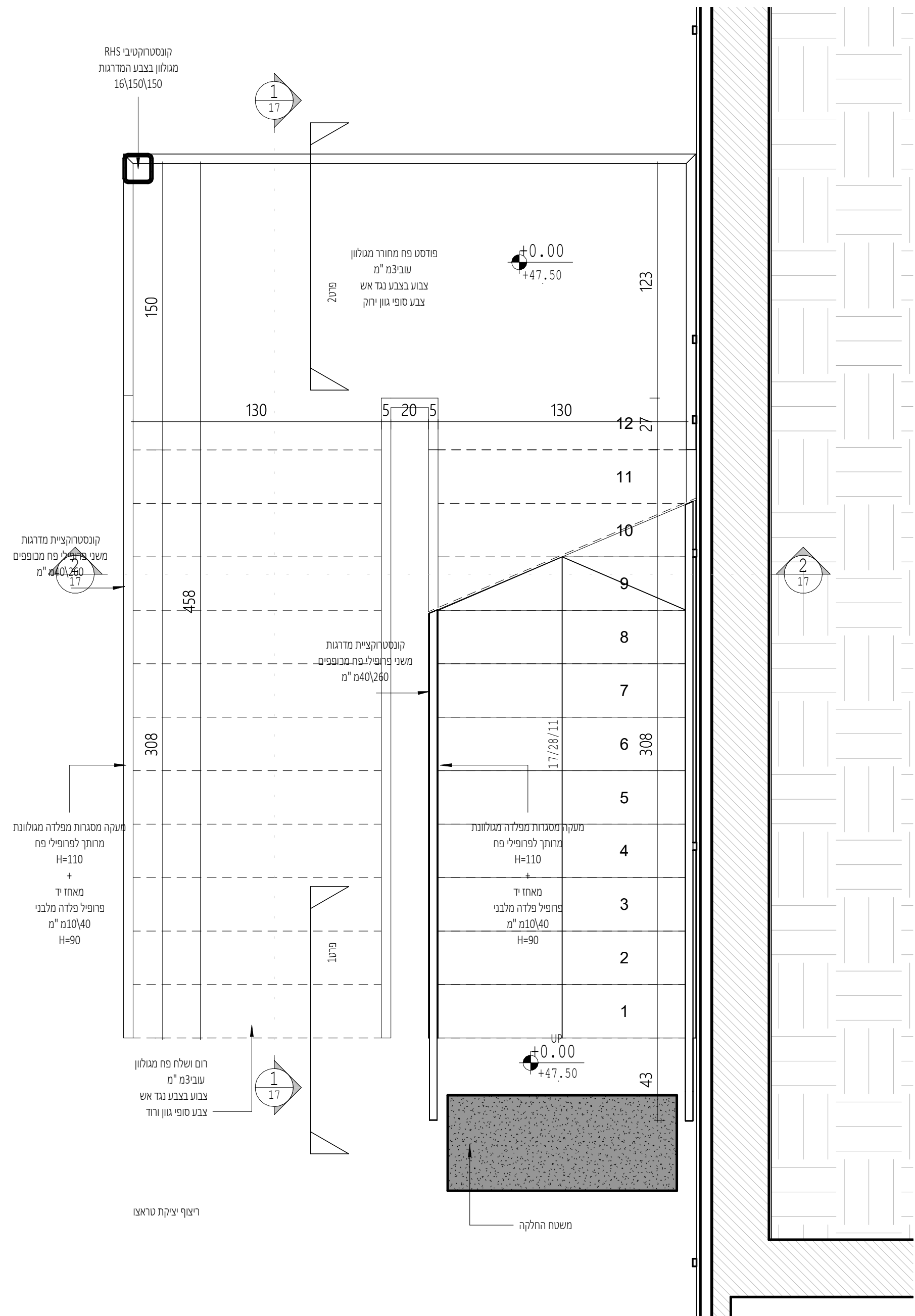
תוכנית קומת קרקע ומדרגות 1 : 20
