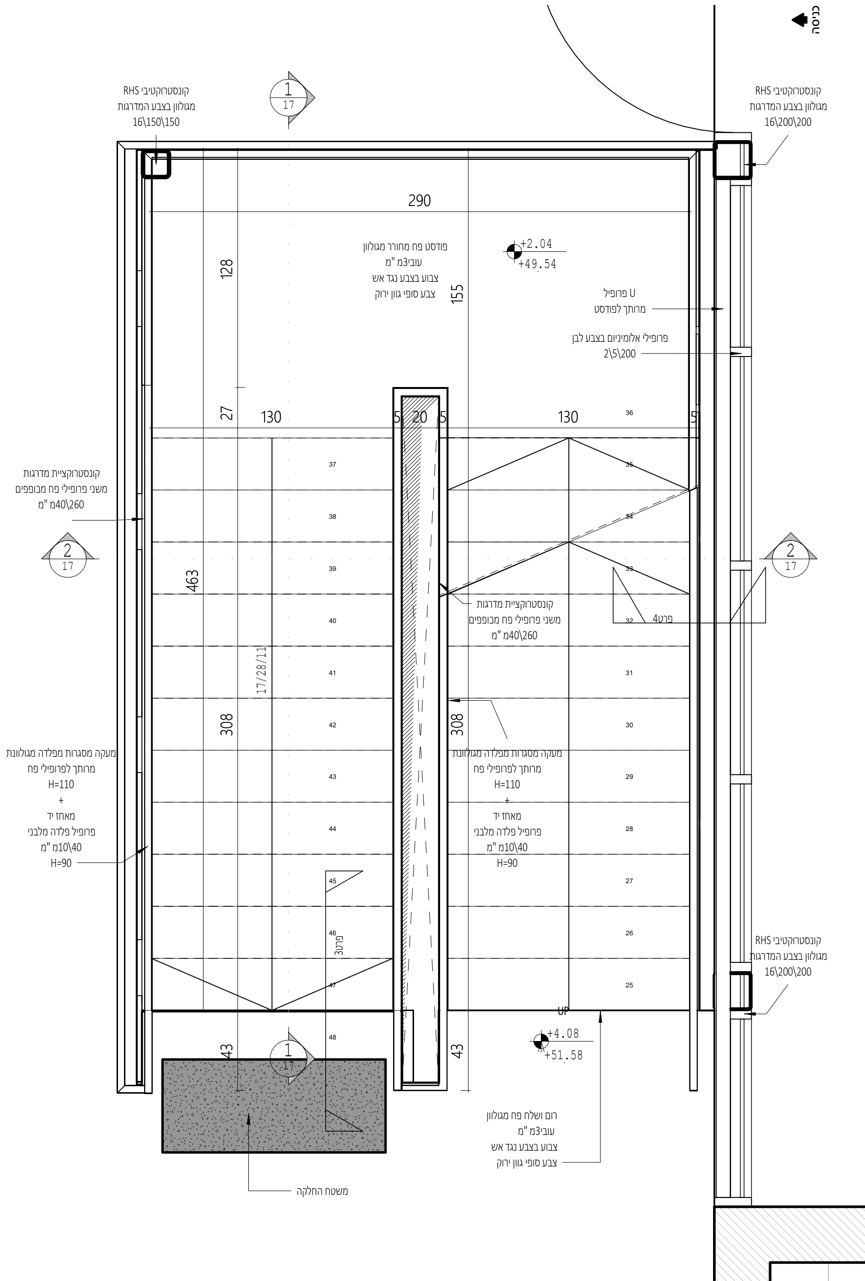
תכנית קומה א ומדרגות 1 : 20
