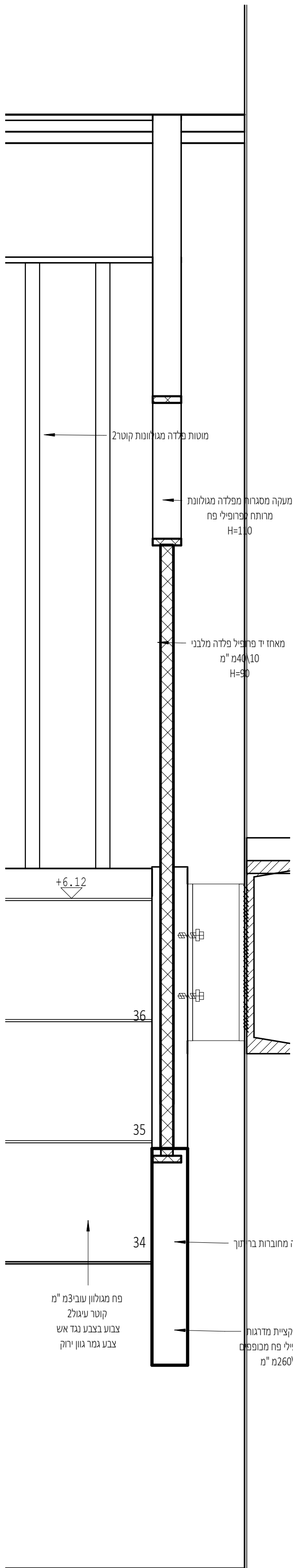
פרט 4 - חיבור מעקה ומדרגות 1 : 5
