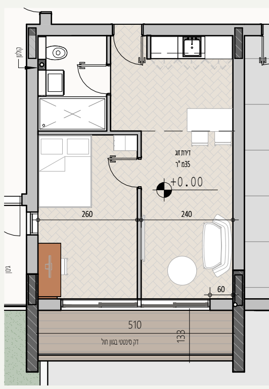
תכנית דירה לזוג 1 : 100
