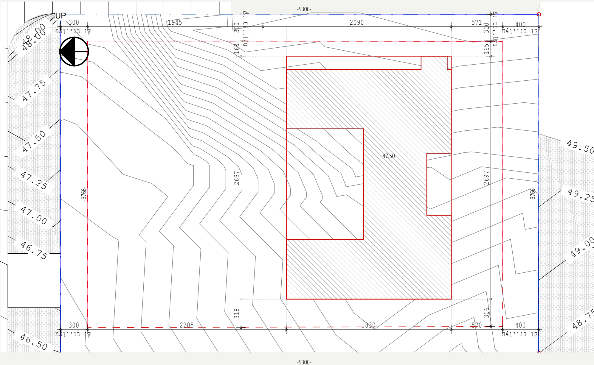
מפה מצבית והעמדה 1 : 250
