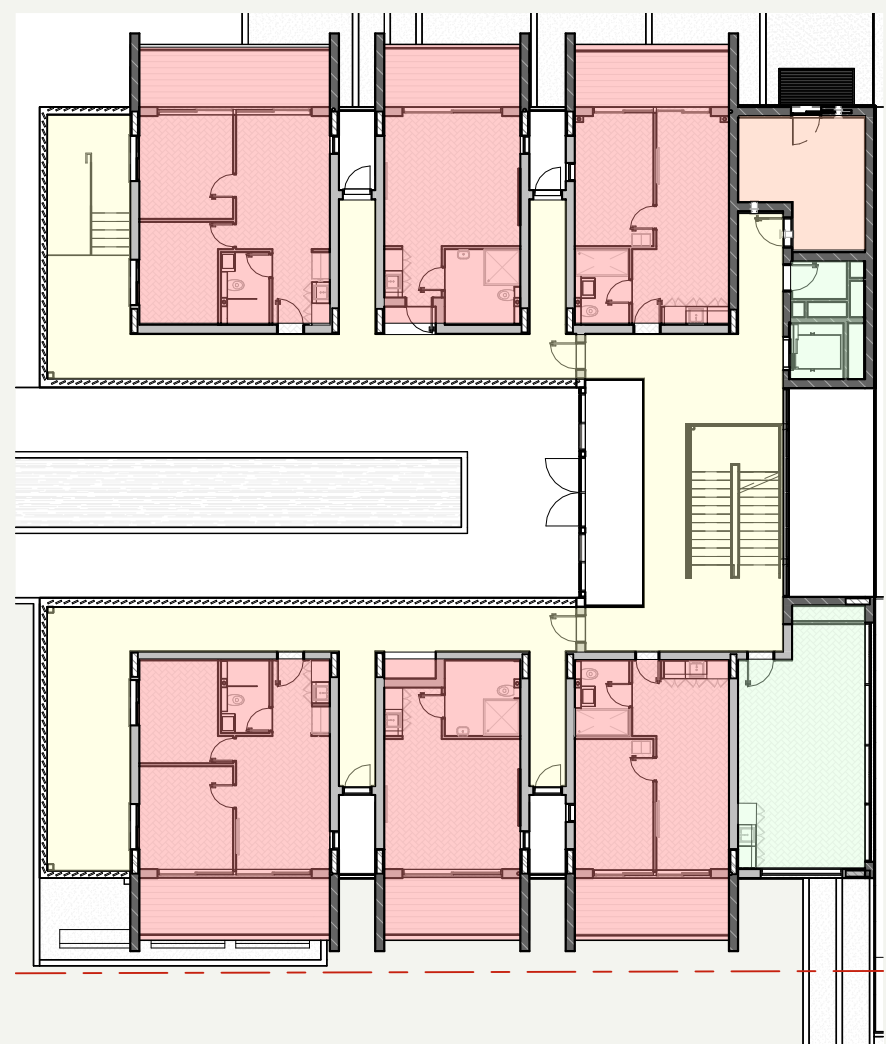
סכמות קומה ב' 1 : 250
