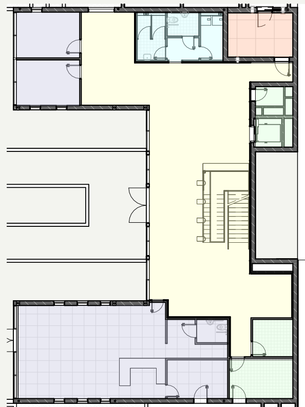
קומת קרקע-סכמות 1 : 250
