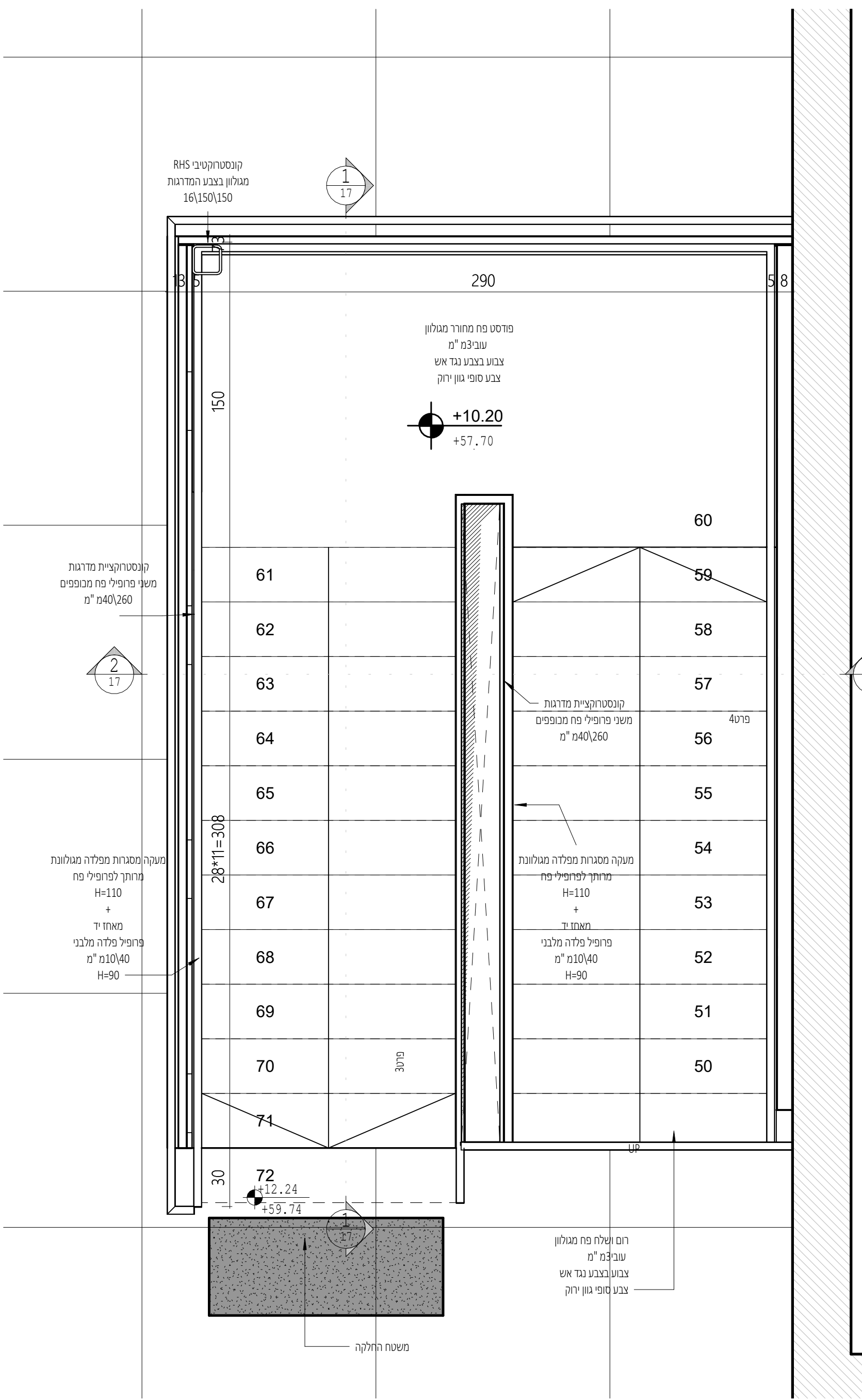
תכנית גג ומדרגות 1 : 20
