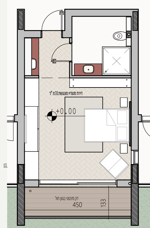
תכנית דירת סטודיו מונגשת 1 : 100
