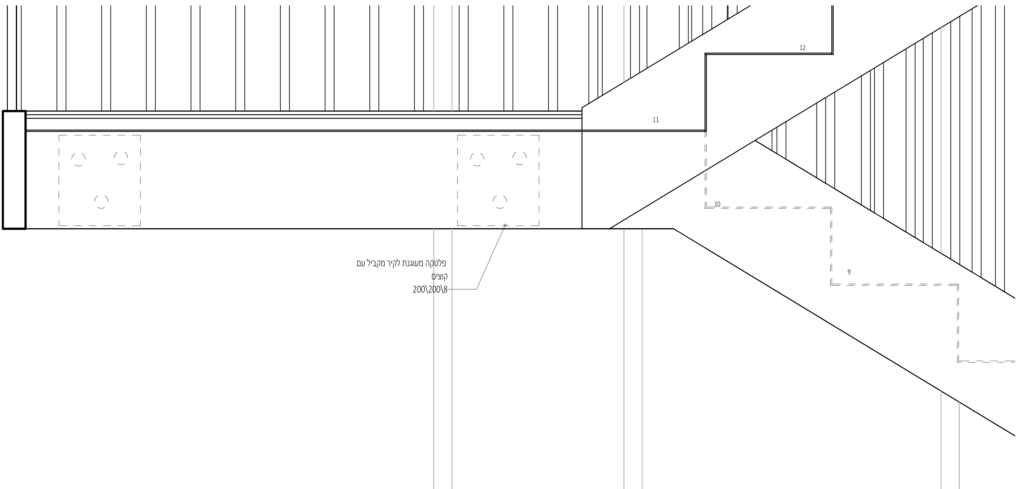
פרט 2 - מדרגות אחרונות 1 : 5
