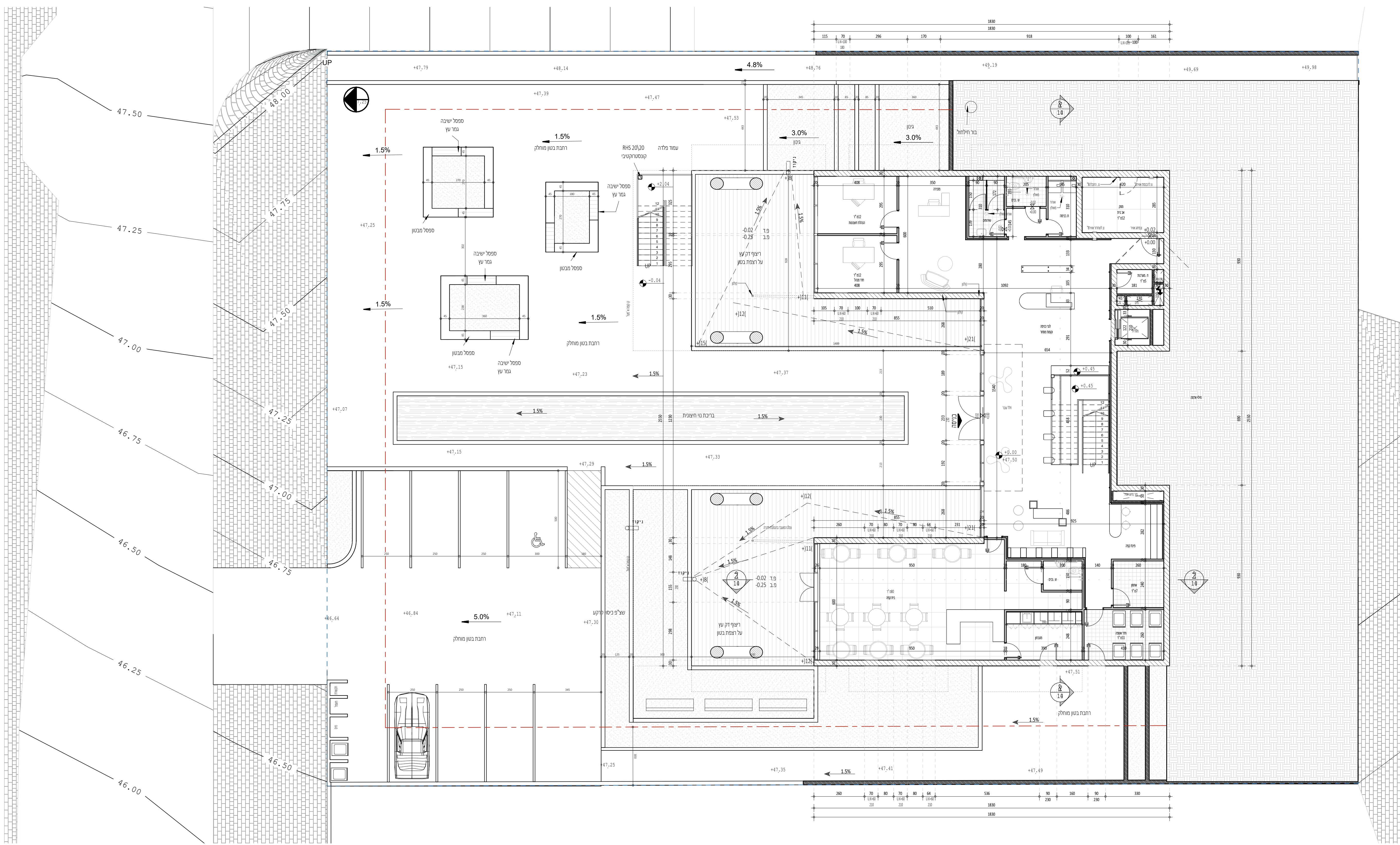
קומת קרקע שחור לבן 1 : 100
