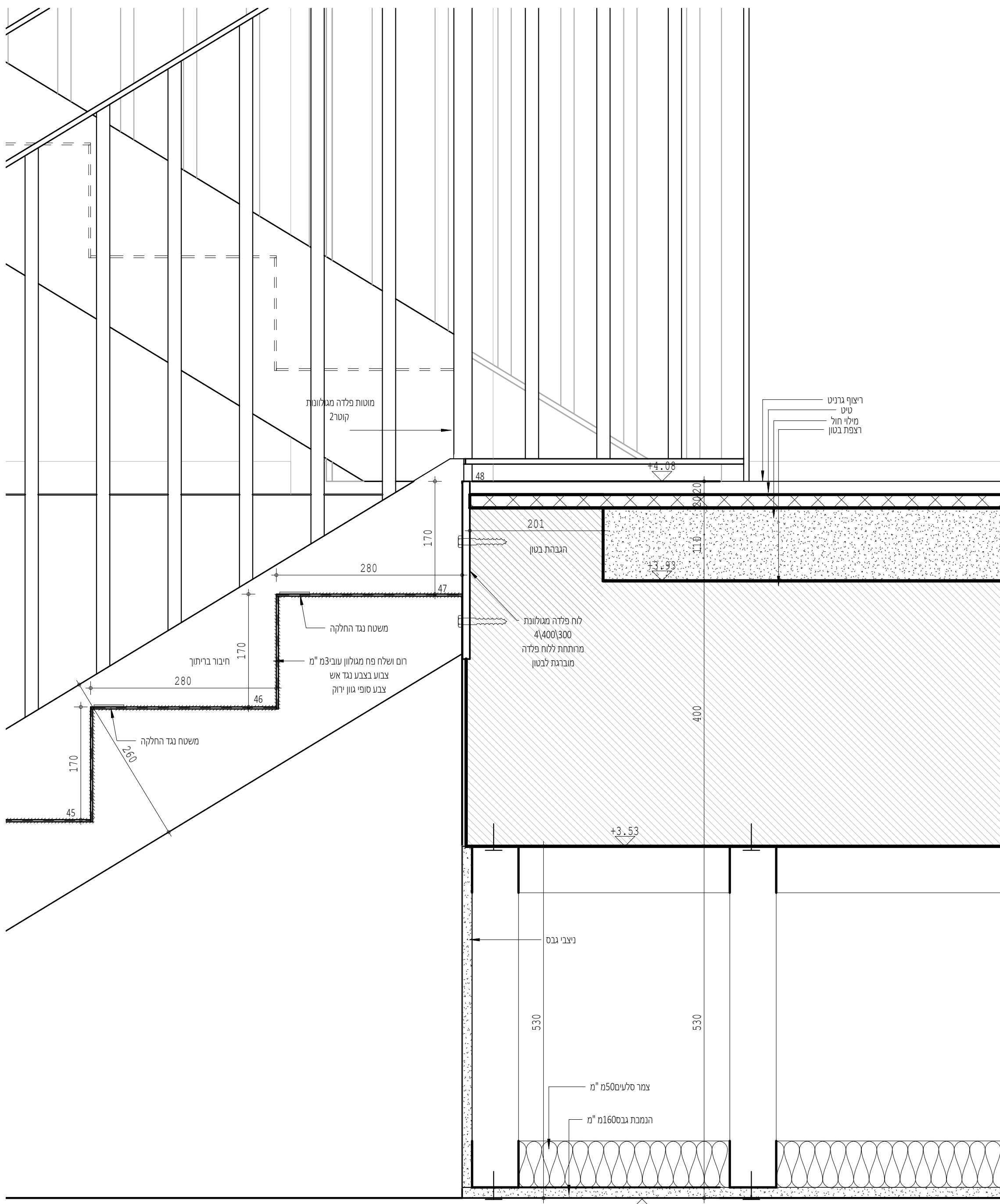
פרט חיבור מדרגה לרצפה 1 : 5
