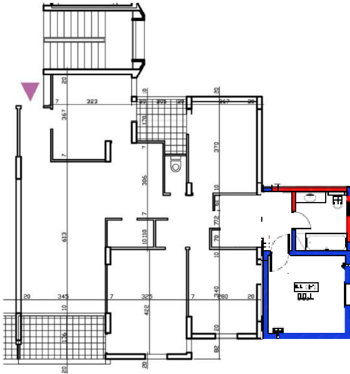
4 חדרים דרום מזרח מצב חדש (כניסה דרך אמבט קיים)
