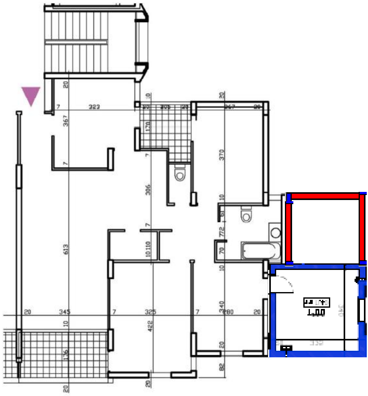
4 חדרים דרום מזרח מצב חדש (כניסה דרך חדר)
