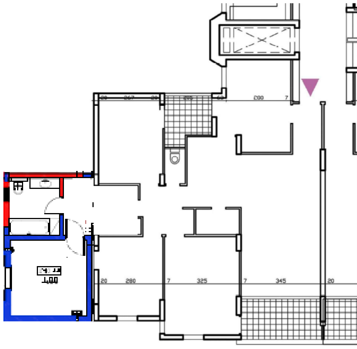
4 חדרים דרום מערב מצב חדש (כניסה דרך אמבט קיים)
