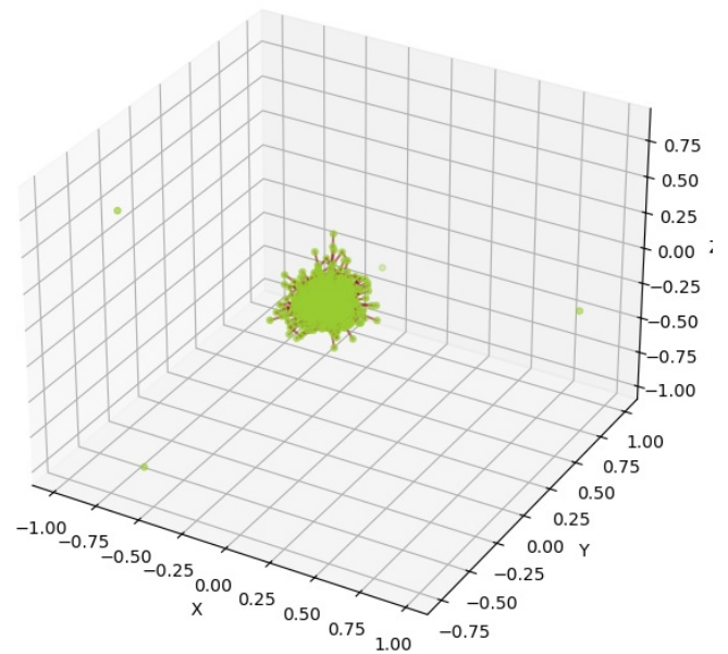
Grafo Nulo Basado en Distancia
