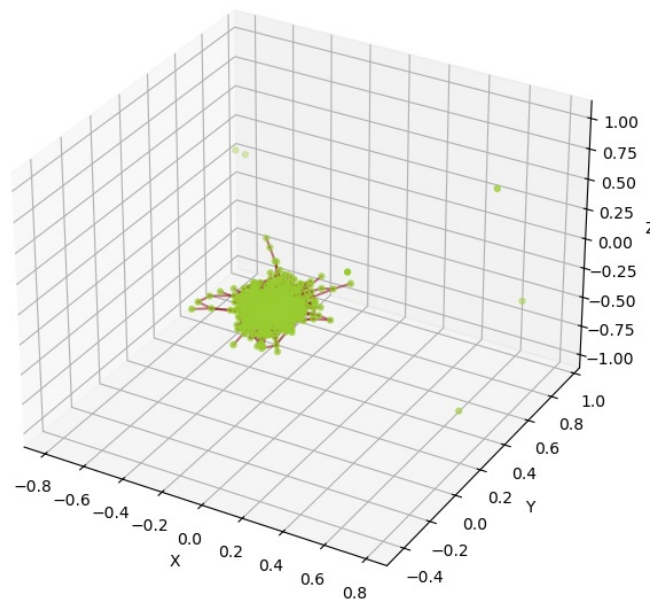
Grafo Nulo Aleatorio
