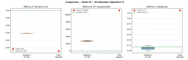
Figure 5: Comportamento comparativo das métricas de robustez sob falhas aleatórias e ataques direcionados.
