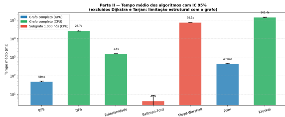
Figure 3: Comparação dos tempos médios de execução com intervalos de confiança de 95% em escala logarítmica.
