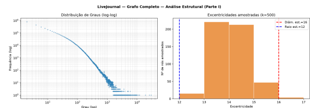
Figure 2: Distribuição de graus em escala log-log (esquerda) e distribuição empírica das excentricidades amostradas (direita).
