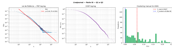
Figure 4: Ajuste de regressão OLS em escala log-log da distribuição empírica de graus.
