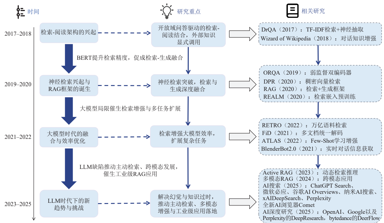
图1 RAG技术发展及研究进展
