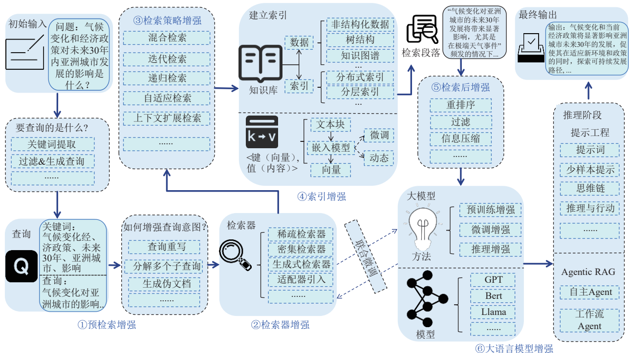
图3 RAG 流程中的增强技术
