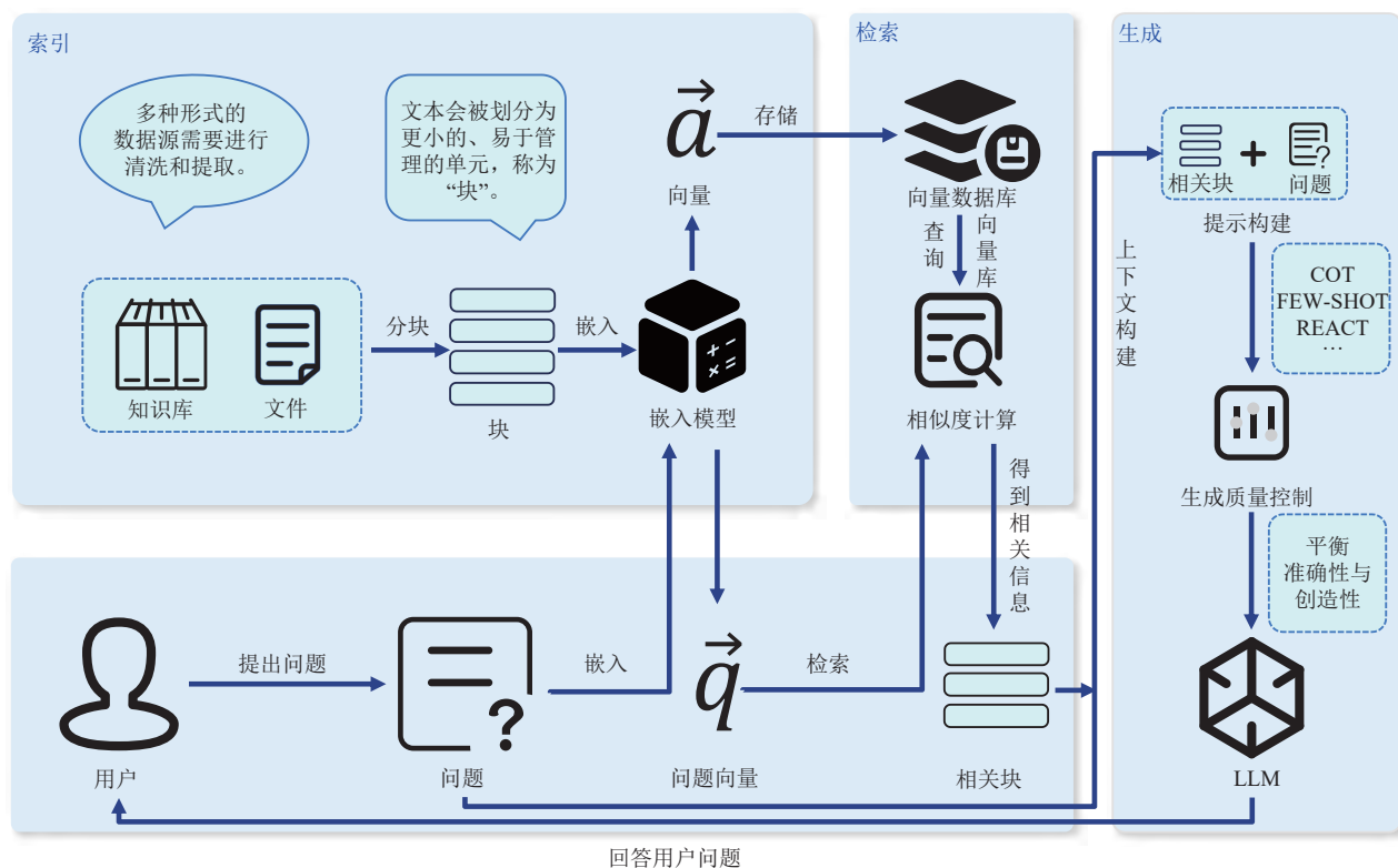
图2 RAG 框架
