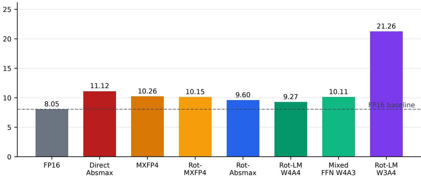
WikiText2 PPL
