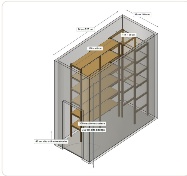
VISTA ISOMÉTRICA
