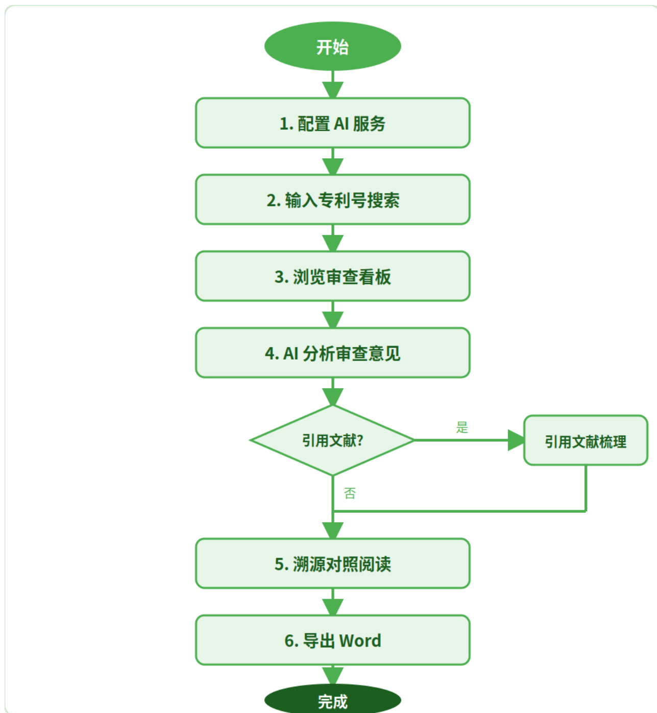
图 7-1 完整操作流程
