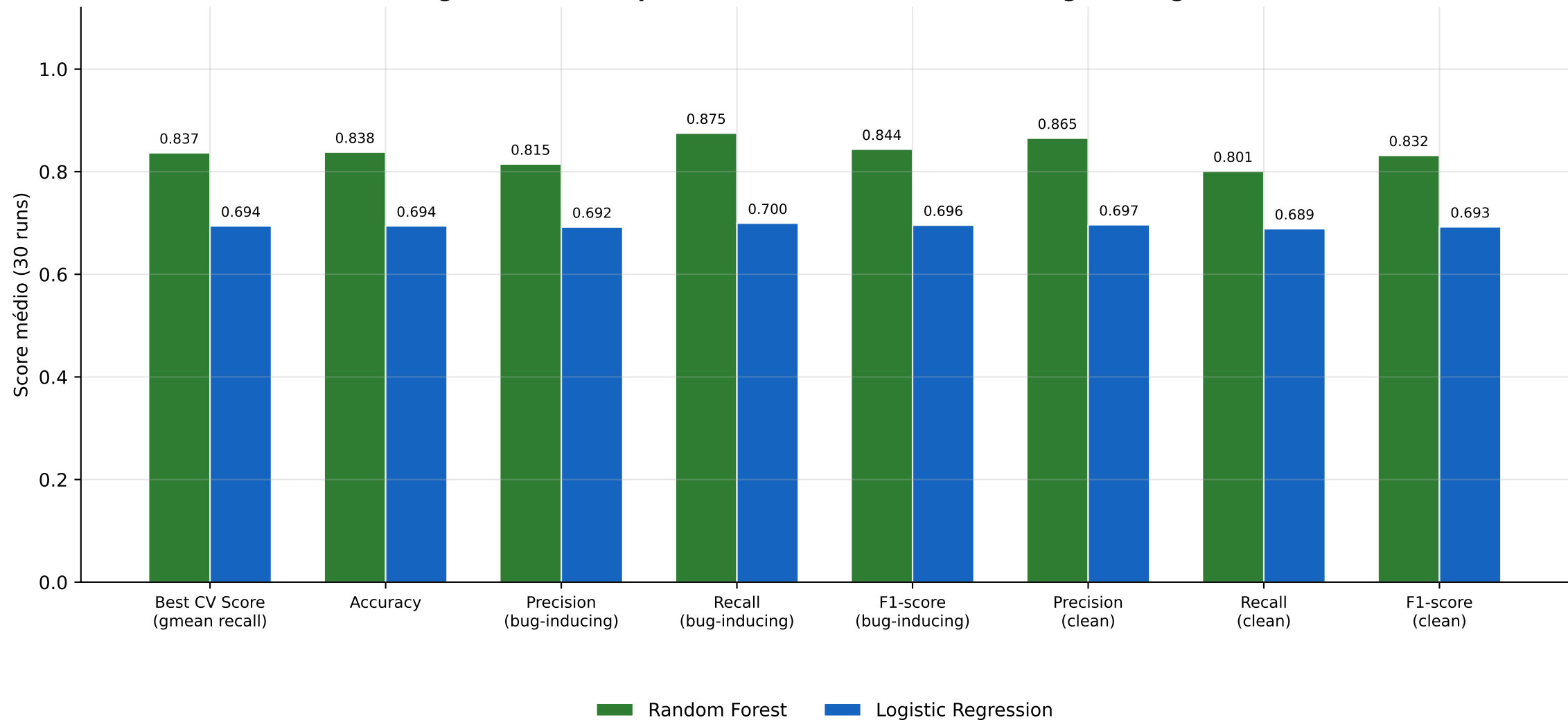
Visão geral — médias por métrica (Random Forest vs Logistic Regression)
