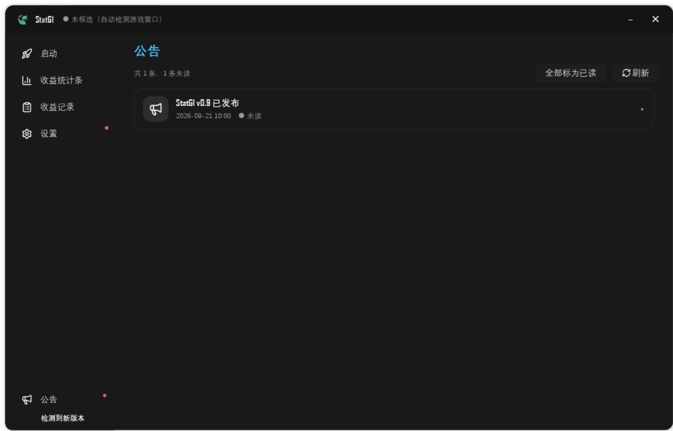
公告页
