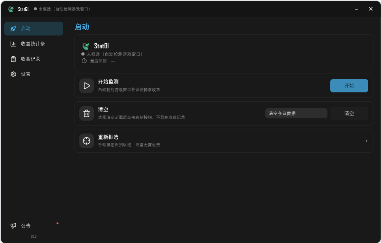
启动页
