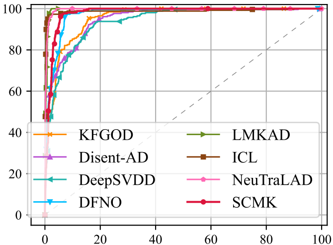
PageBlocks
