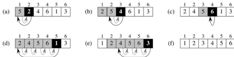
Figur 37: Invarianten i insertionsort: alt til venstre for den nuværende key er altid sorteret.
