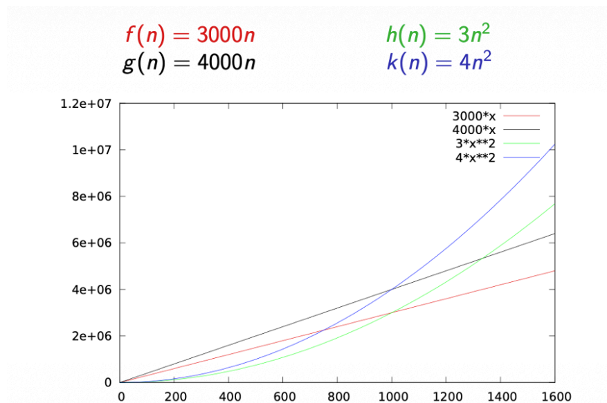
Figur 29: På grafen ser vi at funktionerne h(n) og k(n) altid vil overhale f(n) og g(n) , selvom deres konstant er betydelig mindre.
