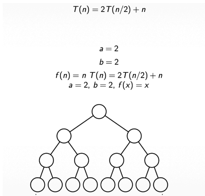
Figur 45: Eksempel: T(n) = 2T(\frac{n}{2}) + n .
