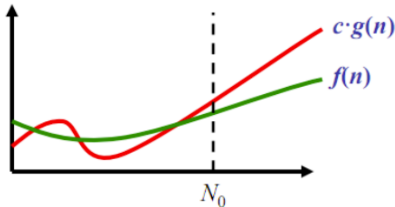
Figur 31: g(n) sætter loftet for hvor hurtigt f(n) må vokse.
