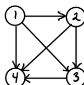
Figur 23: Relationen R_< = \{(a, b) \mid a < b\} på A = \{1, 2, 3, 4\} repræsenteret som matrix og som rettet graf.
