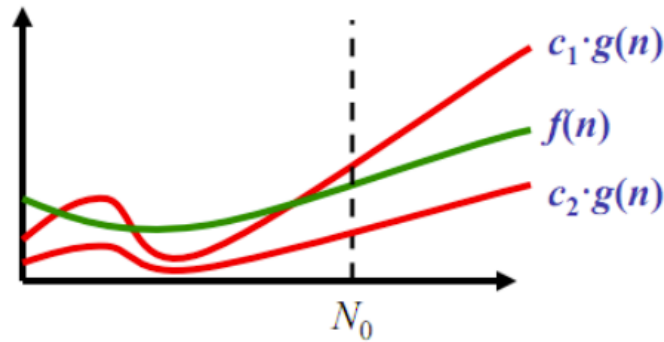
Figur 33: f skal altid ligge mellem de to funktioner med hver sin konstant.
