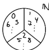
Figur 24: Ækvivalensrelationen a \equiv b \pmod{3} på \mathbb{N} deler mængden i tre ækvivalensklasser [0]_R, [1]_R, [2]_R — en partition af \mathbb{N} . På billedet betyder “mod” modulus.
