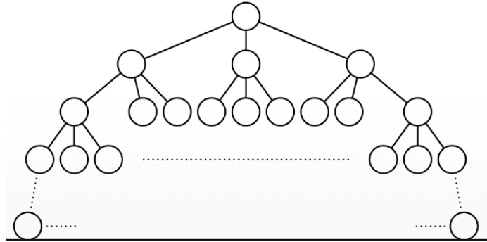
Figur 47: Eksempel 3: T(n) = 3T(\frac{n}{4}) + n^2 .
