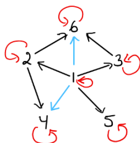
Figur 25: Delelighedsrelationen R = \{(a,b) \mid a \mid b\} på \{1, 2, 3, 4, 5, 6\} . De røde loops følger af refleksivitet, og de blå pile følger af transitivitet.
