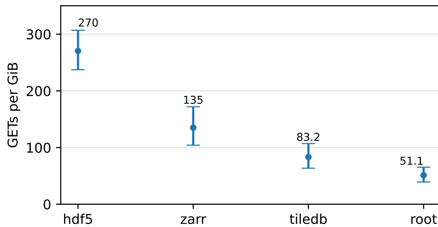
zstd / slice
