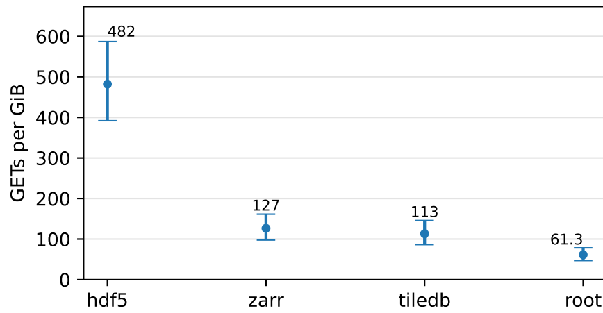
lz4 / slice
