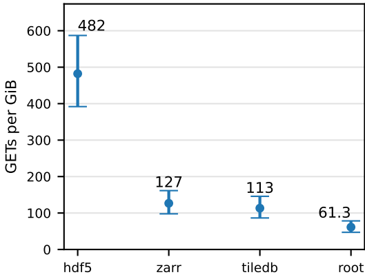
lz4 / slice
