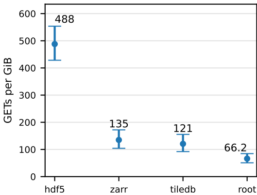
zstd / slice
