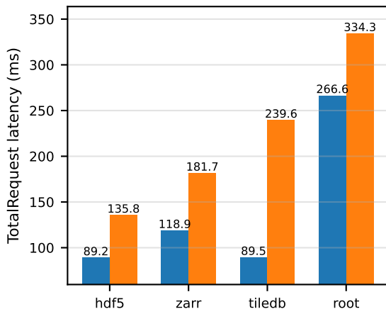
lz4 / slice
