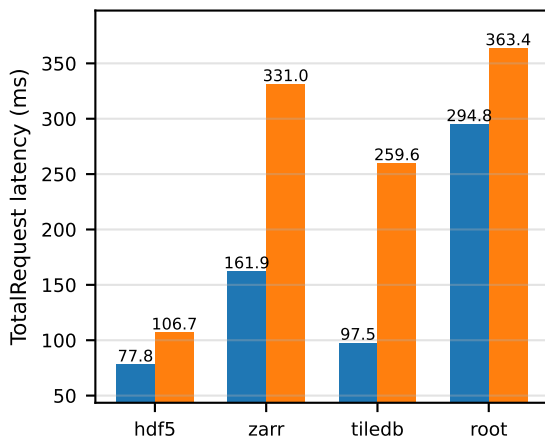
zstd / slice
