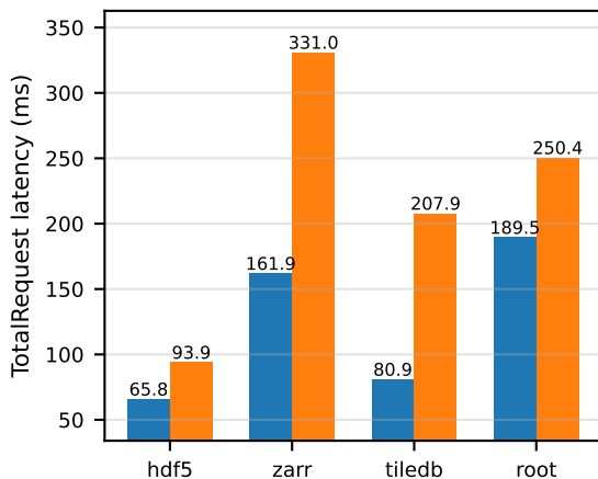
zstd / slice
