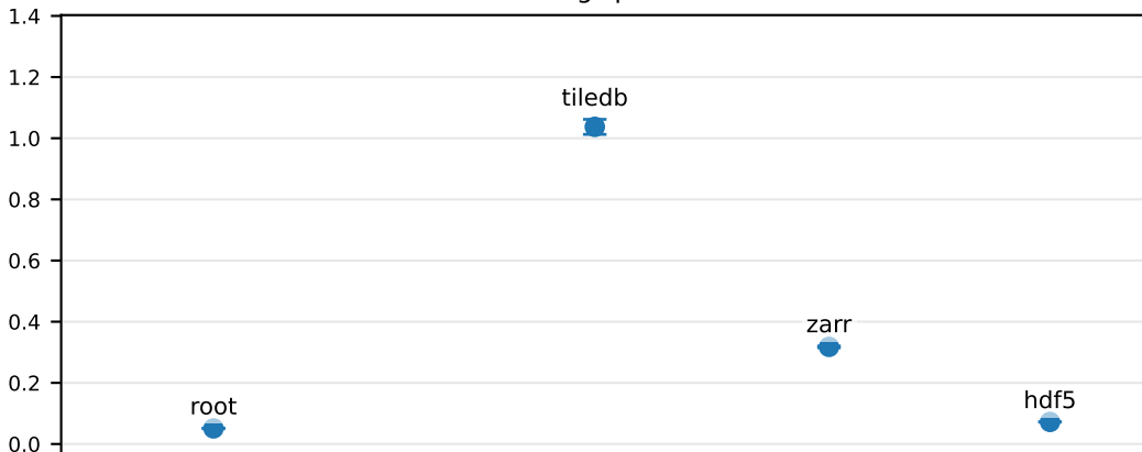
gzip
