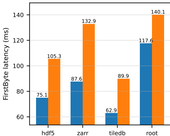
lz4 / slice
