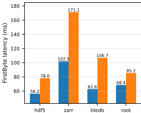
zstd / slice
